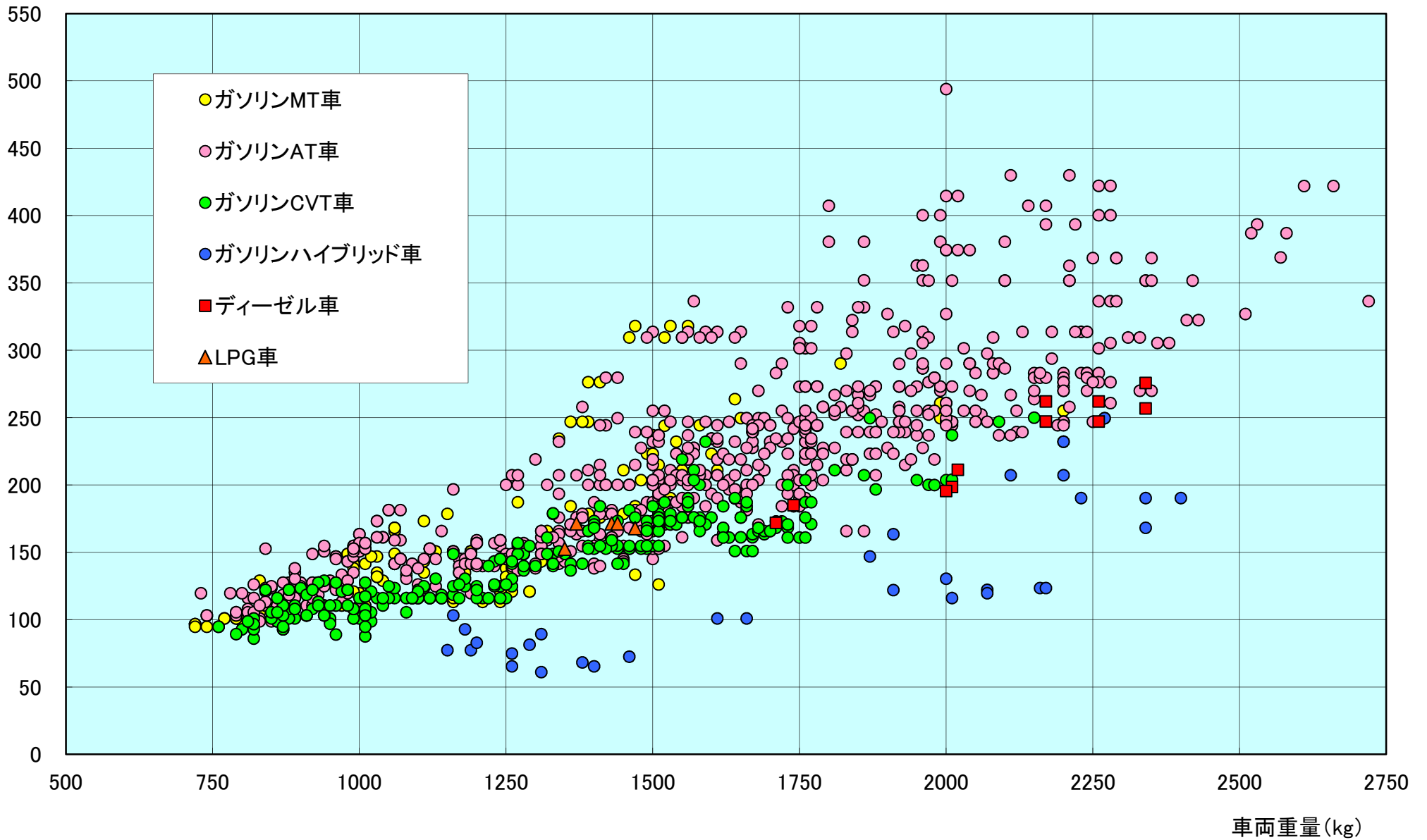
(4) 乗用車 車両重量別CO2排出量(10・15モード)
