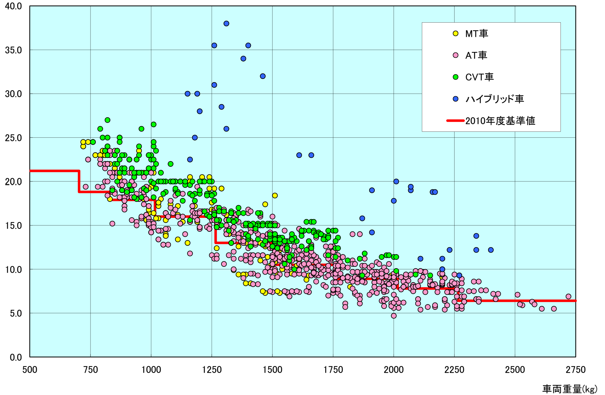
(1)ガソリン乗用車 車両重量別燃費(10・15モード)
