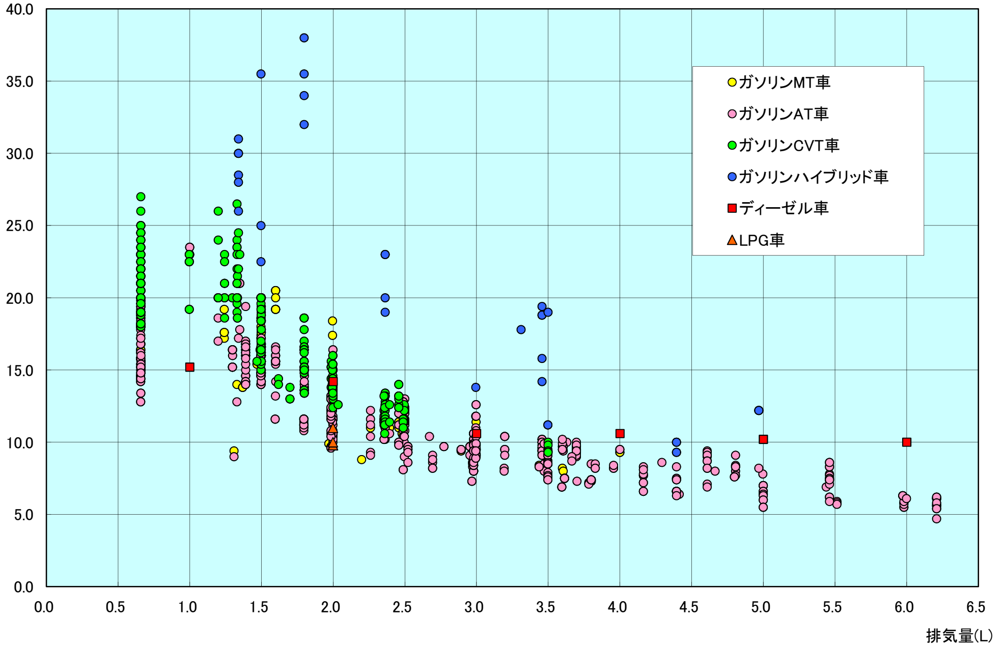
(5) 乗用車排気量別燃費(10・15モード)
