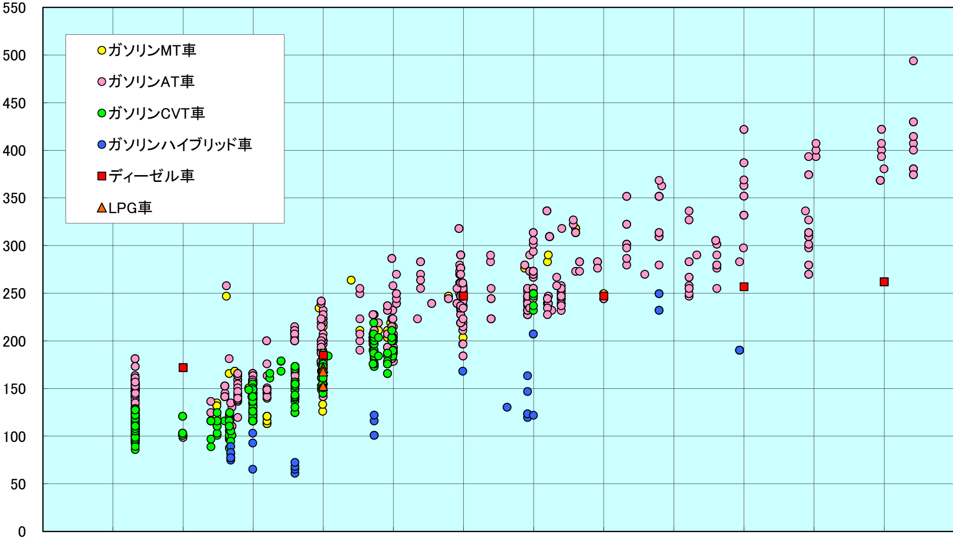
(6) 乗用車排気量別CO2排出量(10・15モード)
