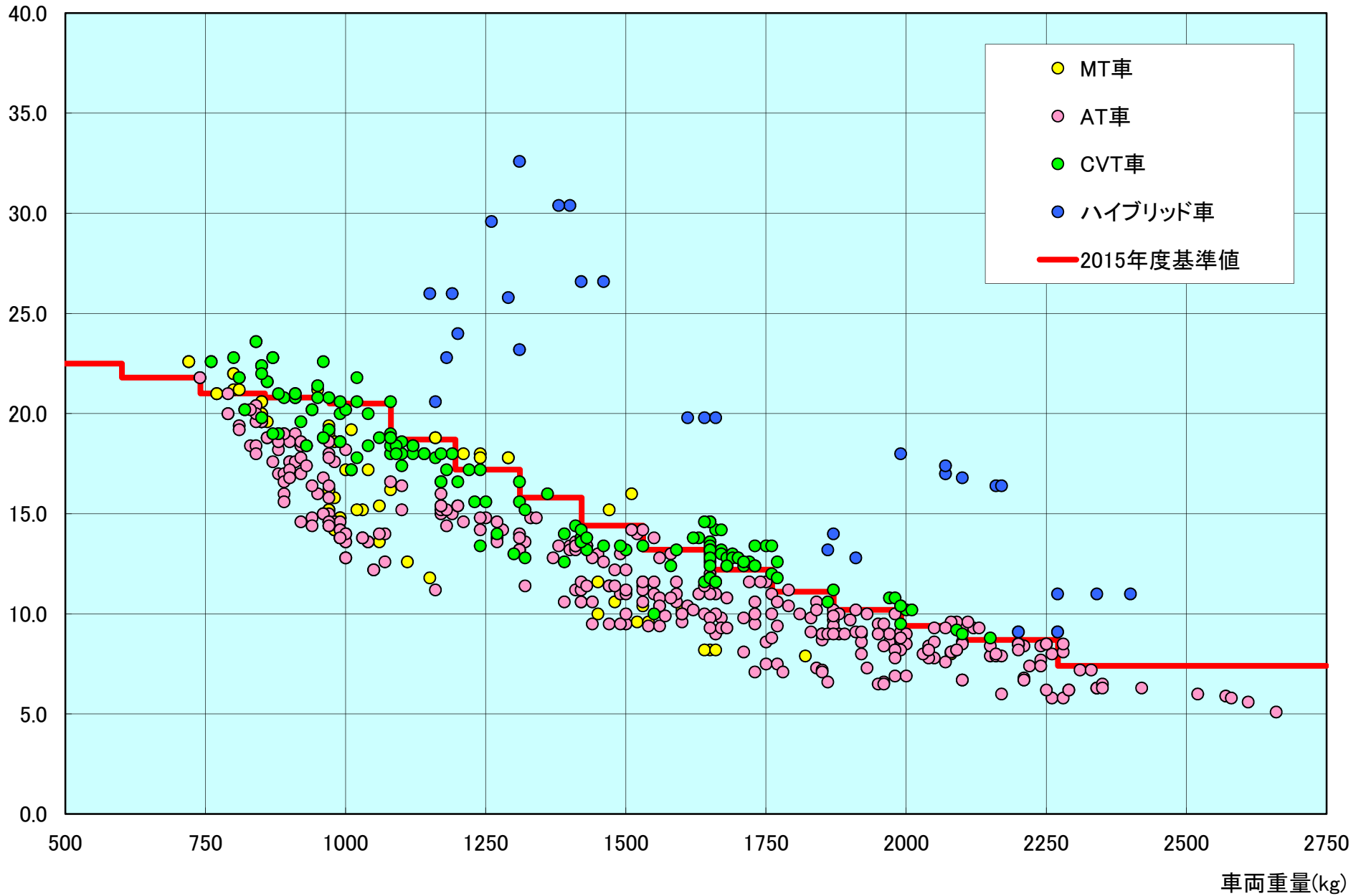
(2)ガソリン乗用車 車両重量別燃費(JC08モード)
