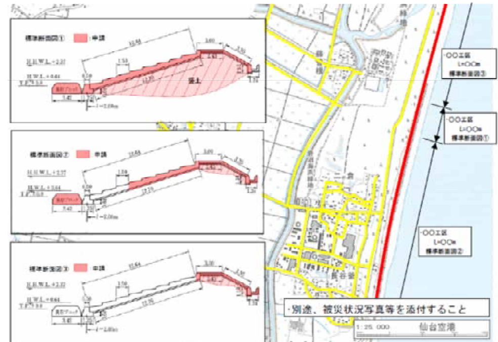
※代表的な被災形態を定め、申請(復旧)計画の標準断面図で設計書を作成。
