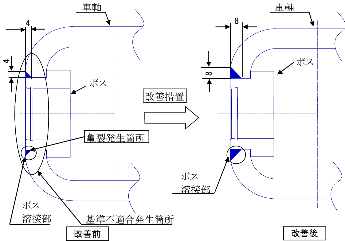
車軸伸縮用シリンダ取付ボス部断面
