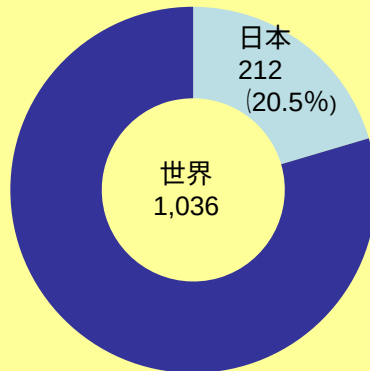
マグニチュード6.0以上の地震回数
