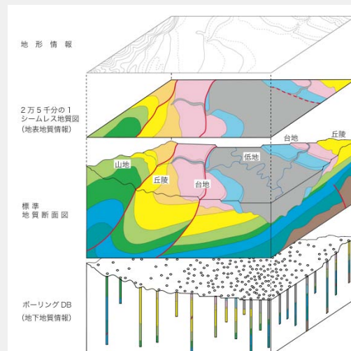
地質情報図(産業技術総合研究所)
