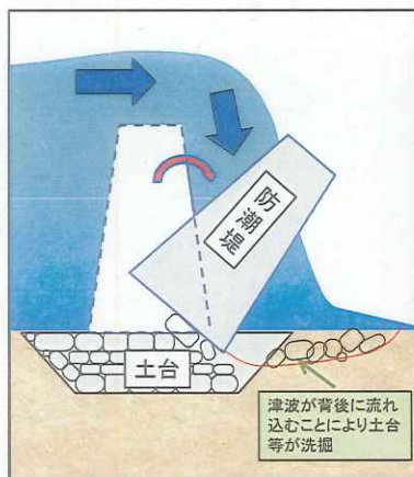
図表7 粘り強い防潮堤のイメージ
