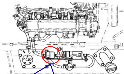
エンジンルーム内
