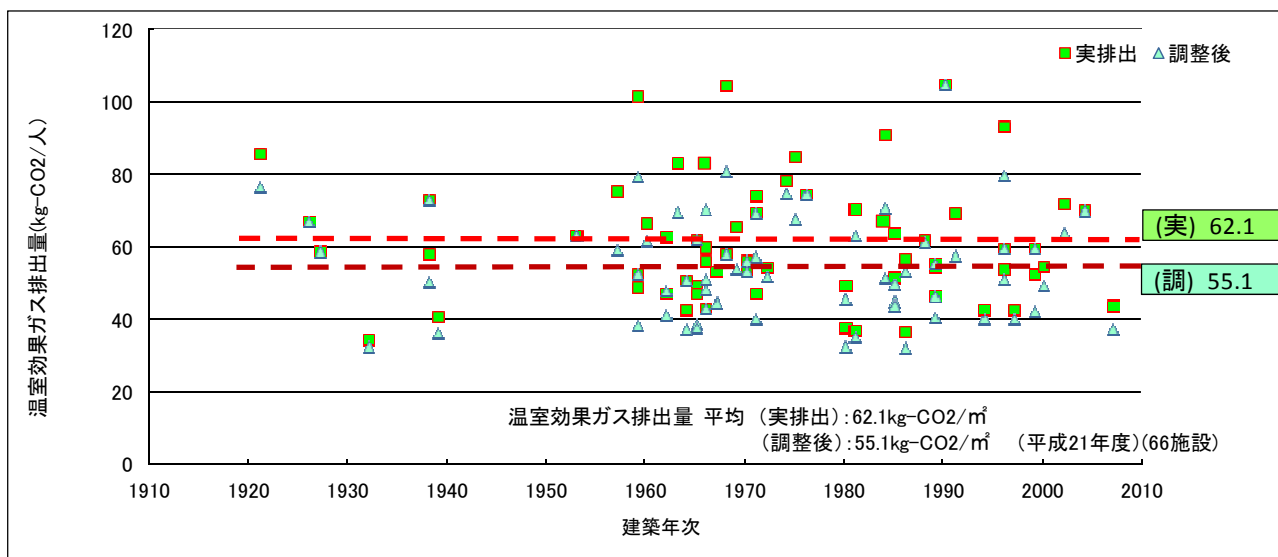
図-9 建築年次と温室効果ガス排出量
