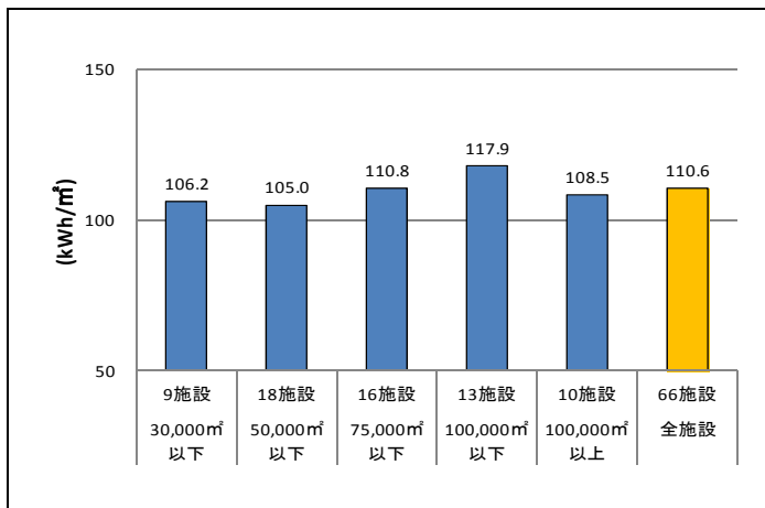
図-14 規模別 単位面積当たり 電気使用量の平均値と施設数(平成 21 年度)
