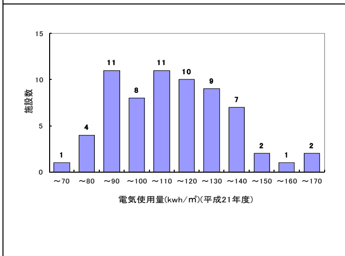
図-19 単位面積当たりの電気使用量と施設数
