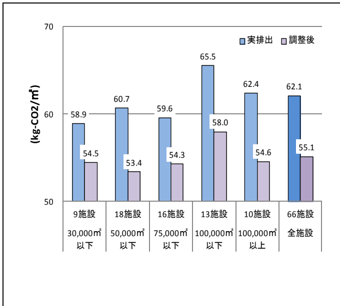
図-7 規模別 単位面積当たり 温室効果ガス排出量の平均値と施設数(平成 21 年度)
