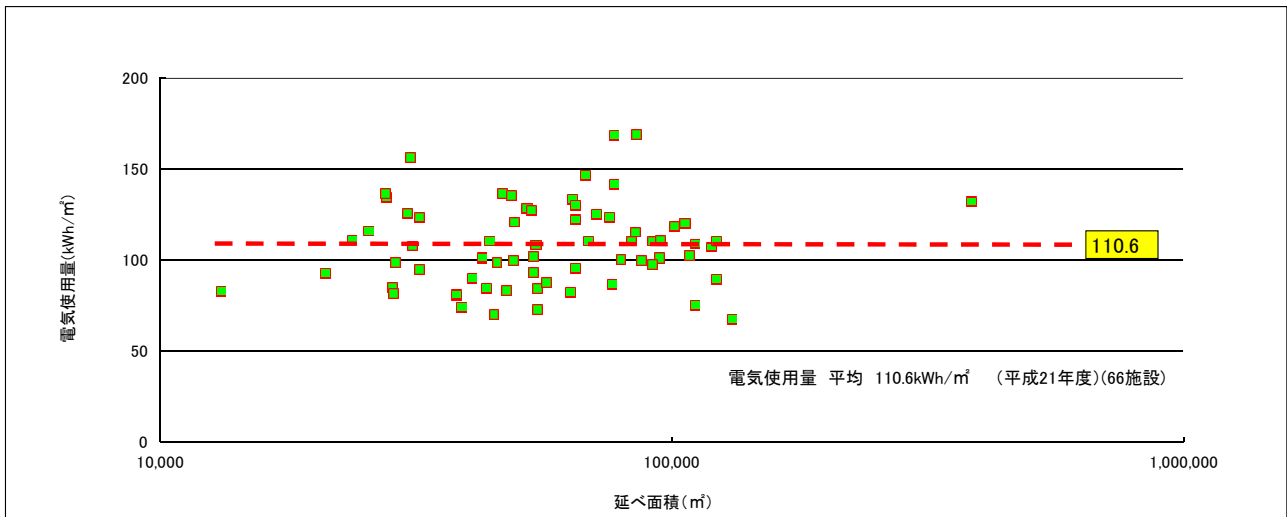
図-12 延べ床面積と電気使用量
