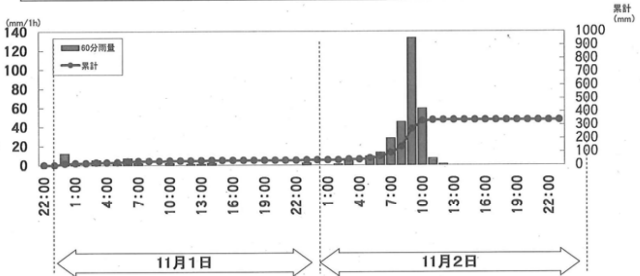
瀬戸内町古仁屋地域気象観測所(アメダス)での雨量データ(気象庁雨量計)
