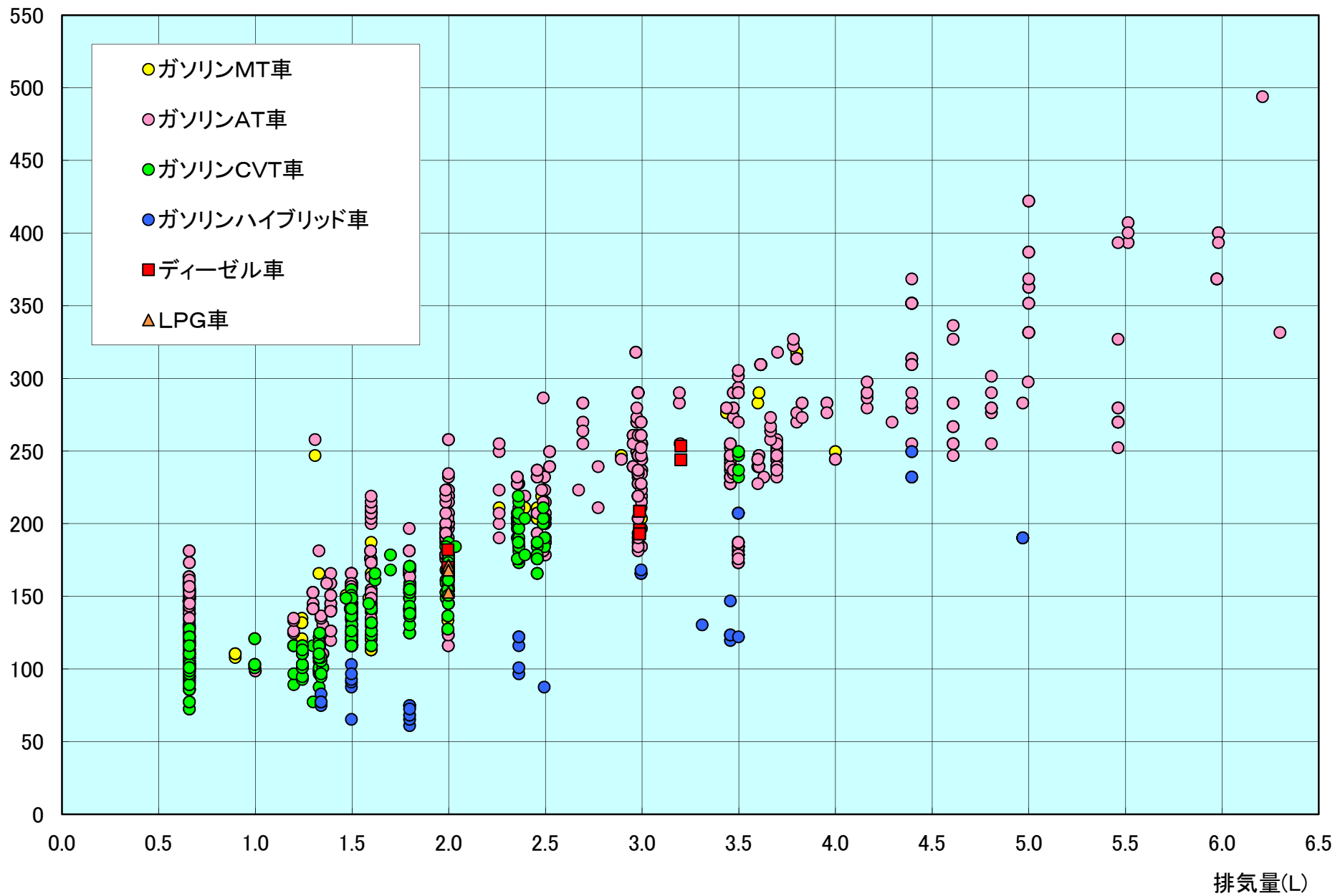
(6)-2 乗用車 排気量別CO2排出量(10・15モード)
