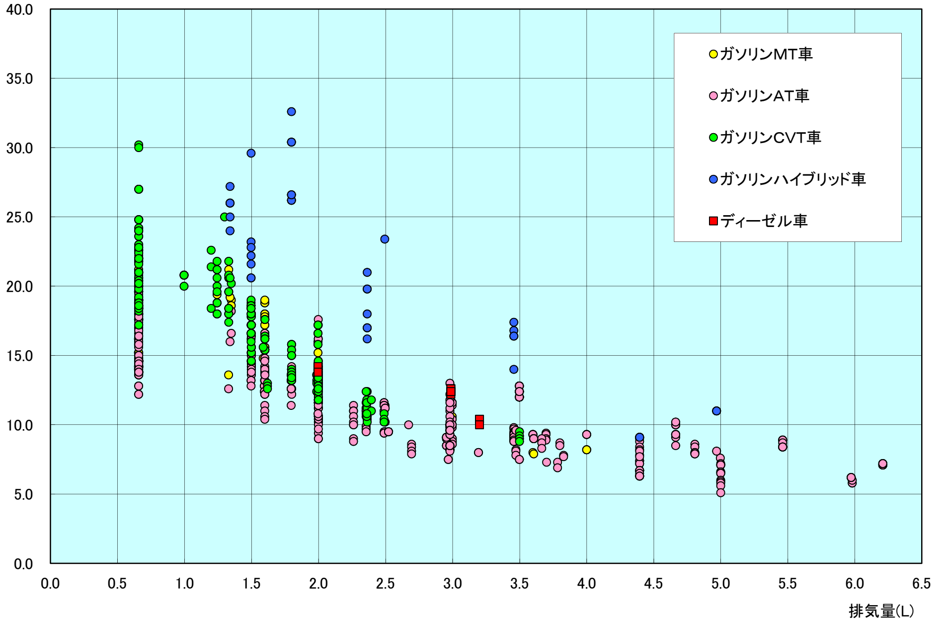
(5)-1 乗用車 排気量別燃費(JC08モード)
