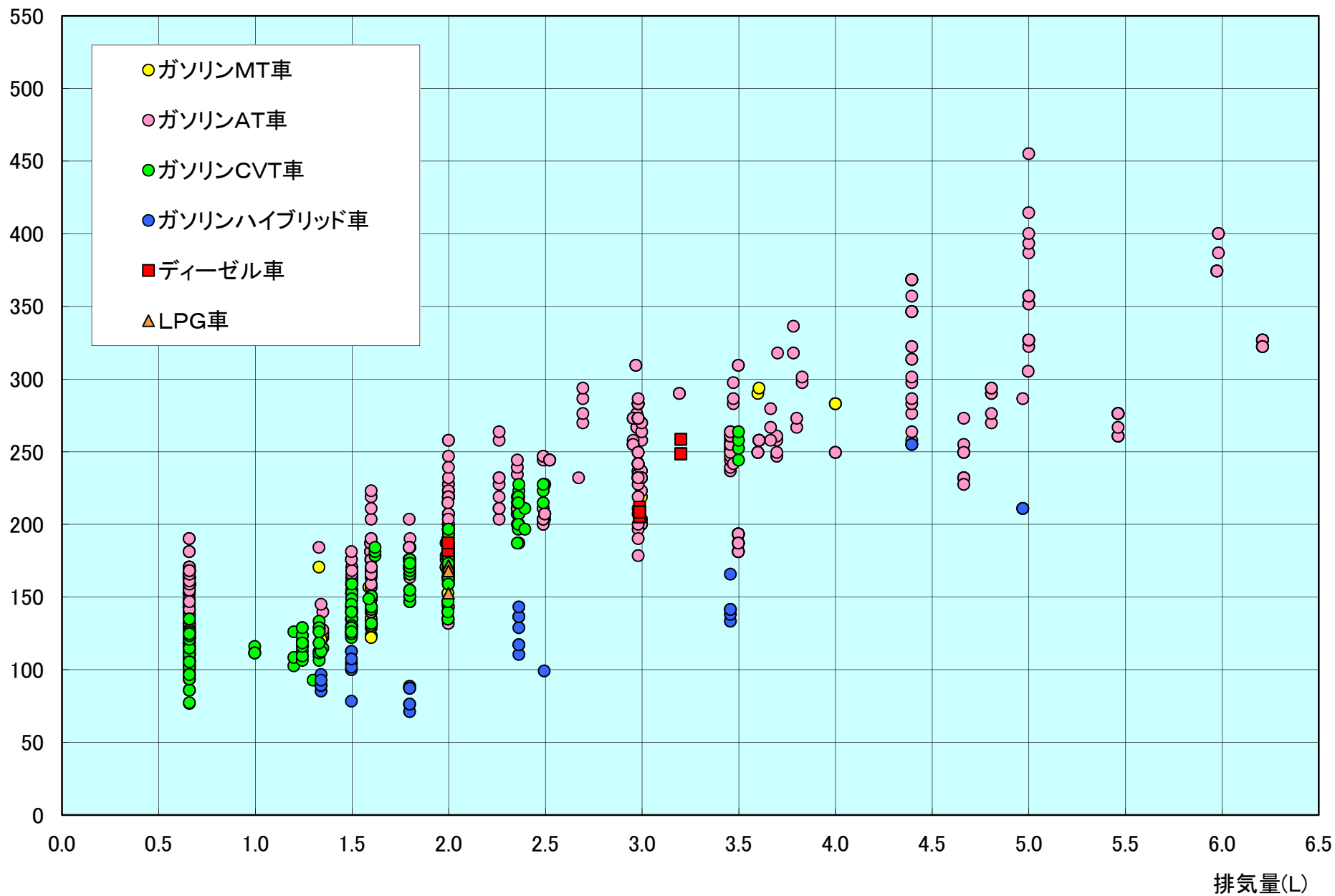
(6) - 1 乗用車 排気量別CO2排出量(JC08モード)
