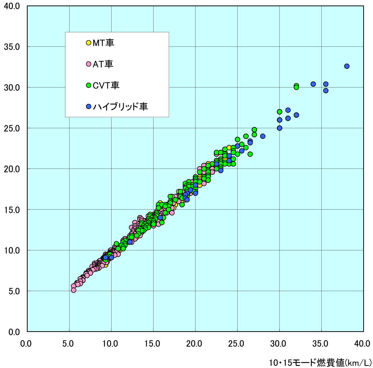
(3)ガソリン乗用車 10・15モード燃費値と JC08モード燃費値との関係
