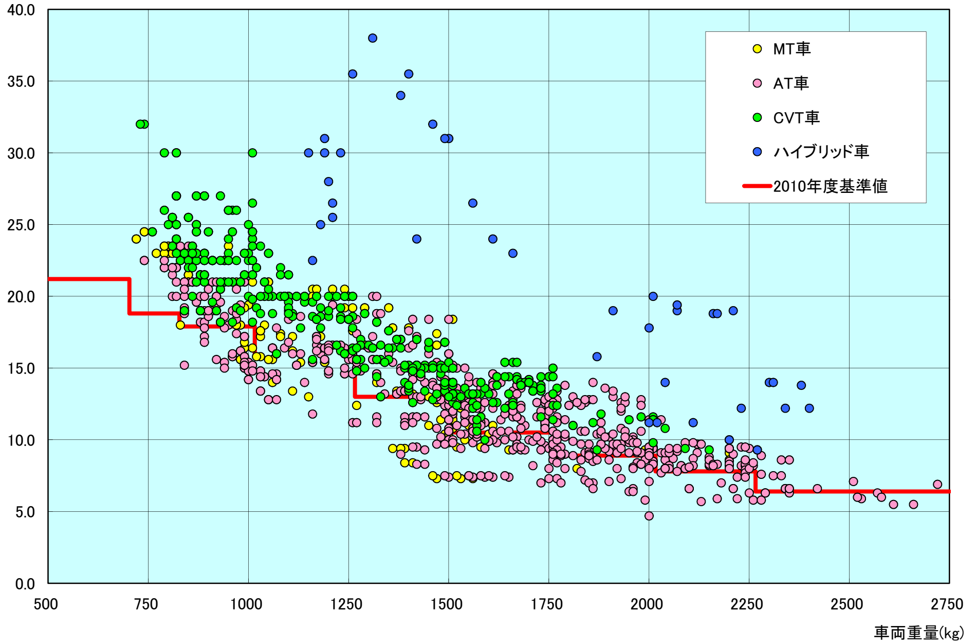
(2)ガソリン乗用車 車両重量別燃費(10・15モード)
