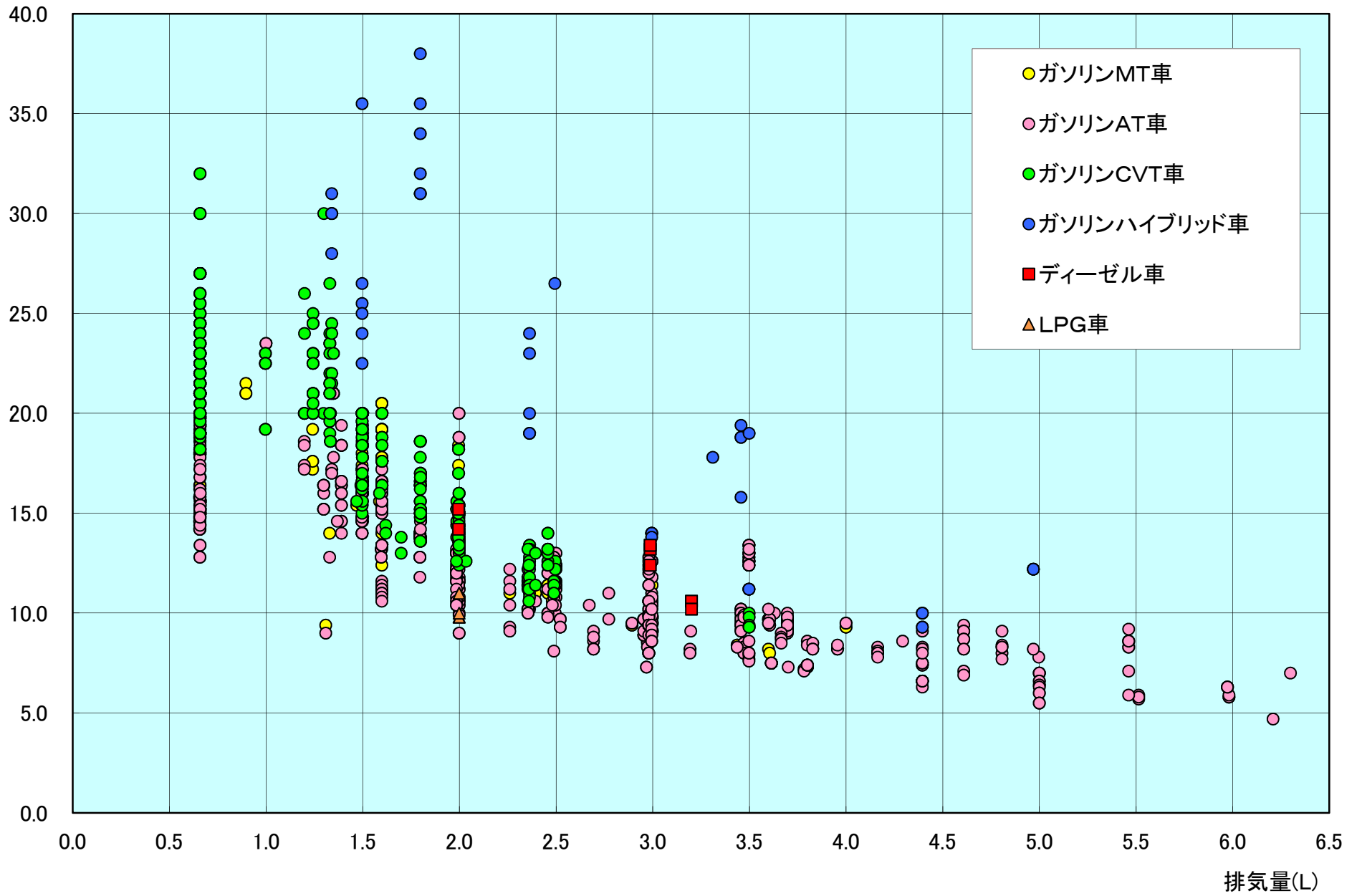
(5) - 2 乗用車 排気量別燃費(10・15モード)
