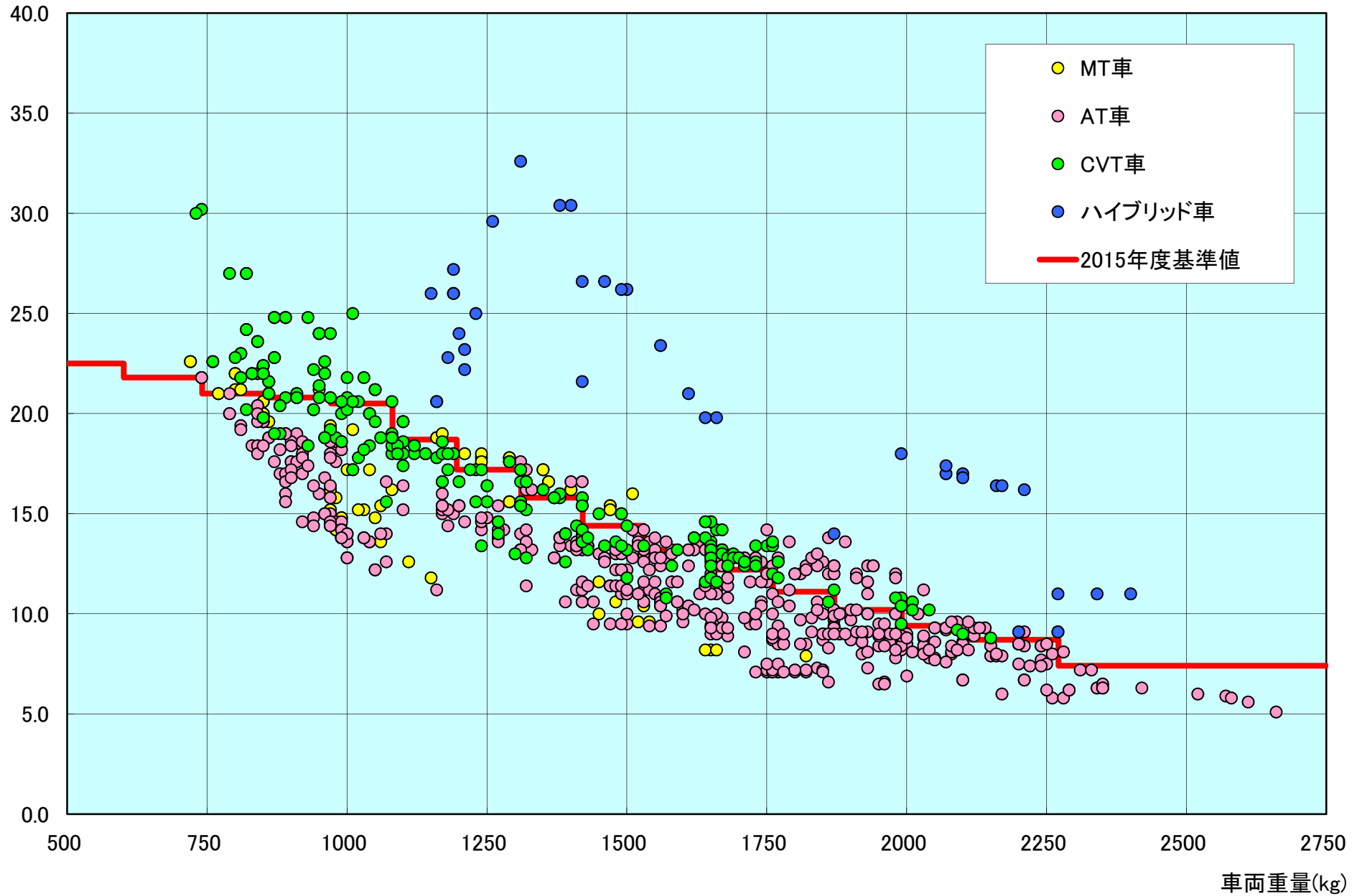
(1) ガソリン乗用車 車両重量別燃費(JC08モード)
