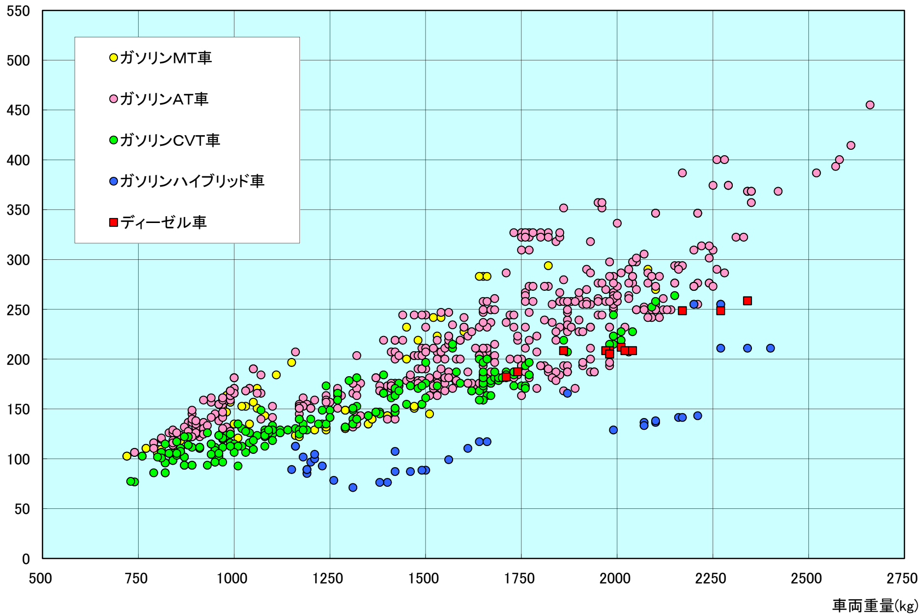
(4) - 1 乗用車 車両重量別CO2排出量(JC08モード)
