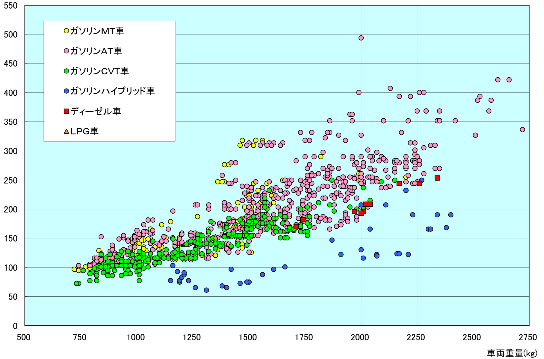
(4)-2 乗用車 車両重量別CO2排出量(10・15モード)
