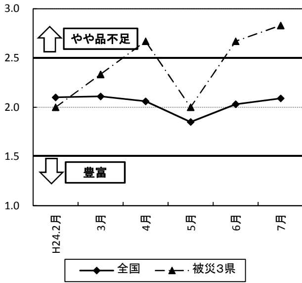
骨材(砂)
