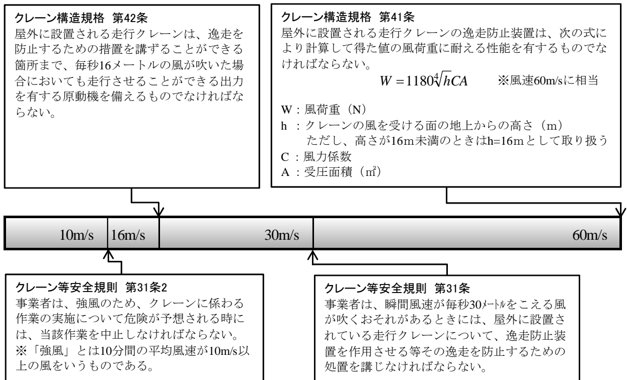
図-3.4.1 クレーンにおける風速規定
