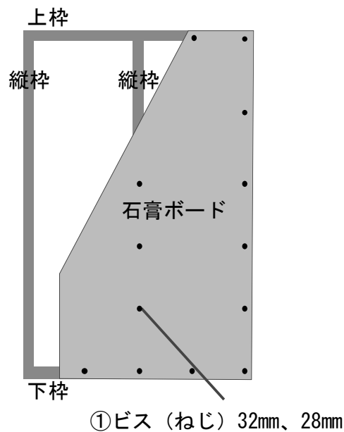
図1. 間仕切壁 (イメージ)
