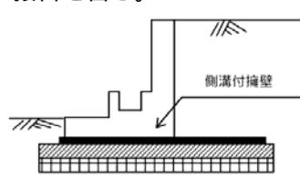
側溝付プレキャスト擁壁の例
