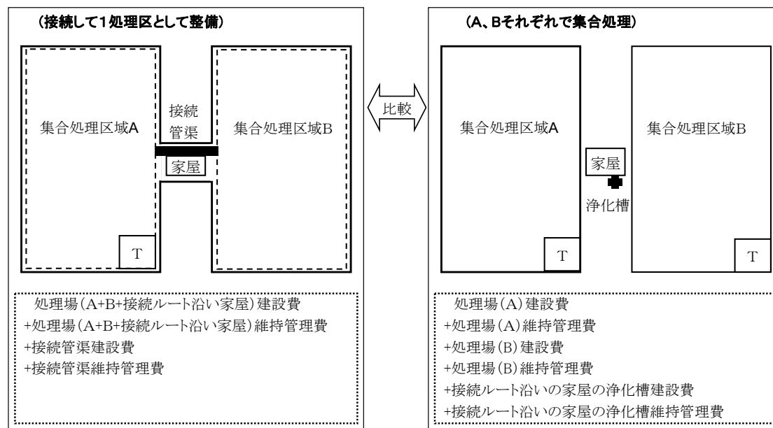
(既整備区域等と他の集合処理区域の接続検討 (イメージ))
