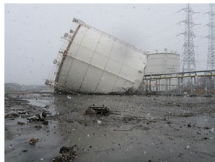
被災したガスホルダー（仙塩浄化センター）
