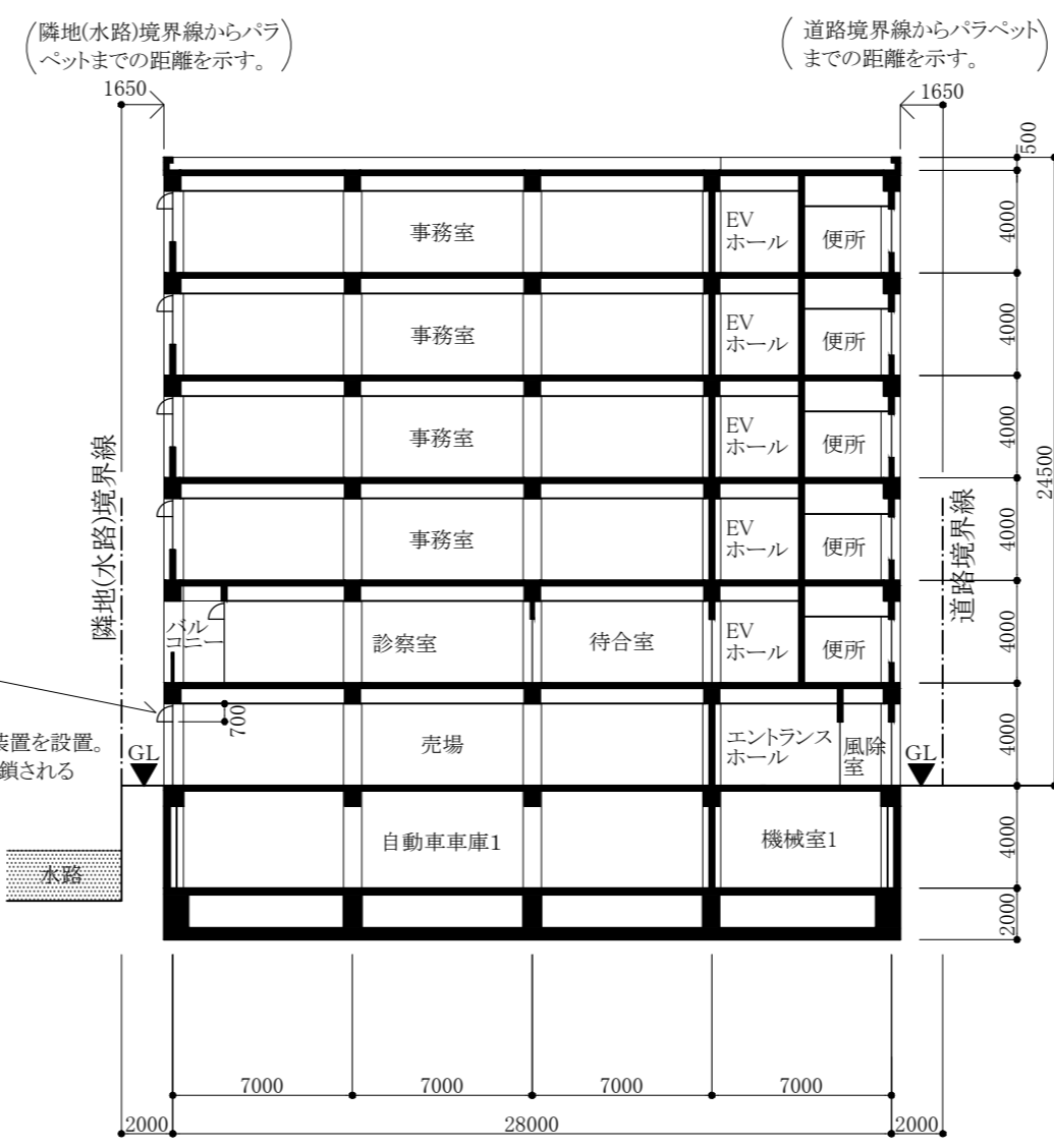
A-A' 断面図
