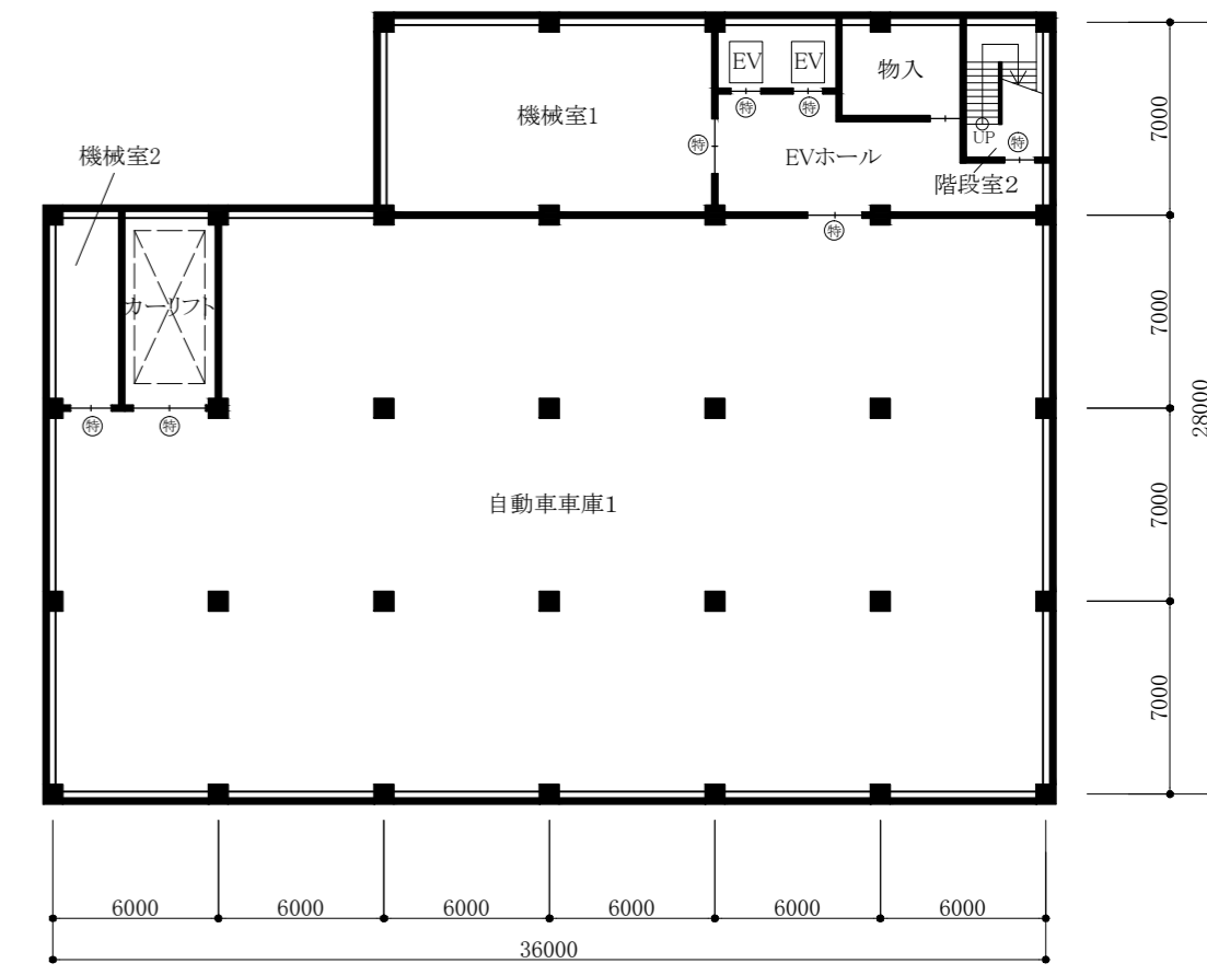
地下1階平面図
