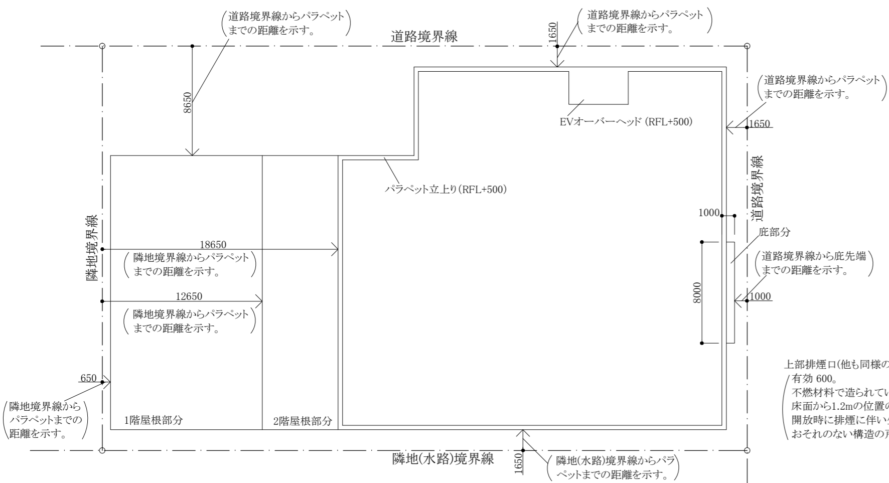
屋上階平面図
