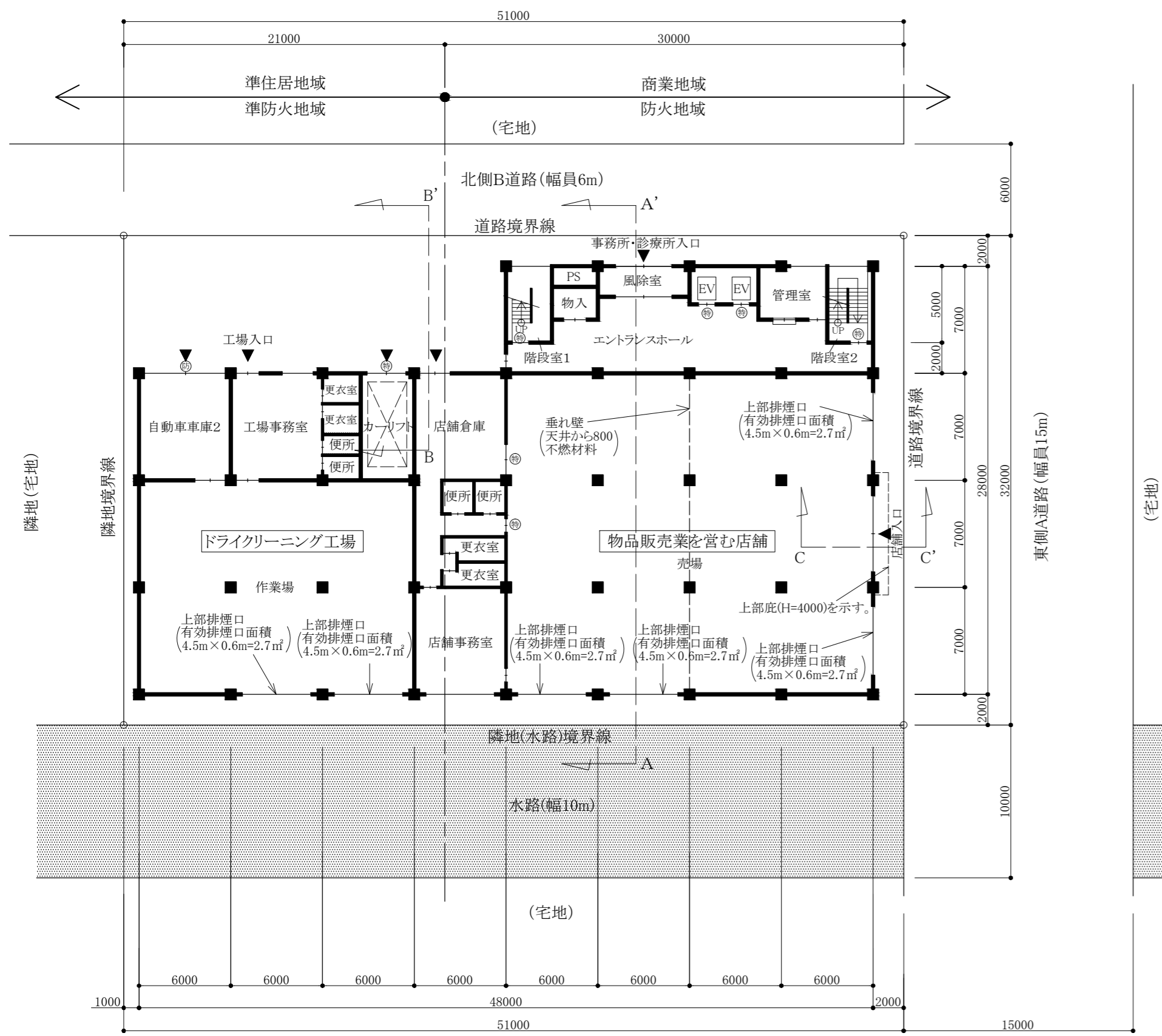
1階平面図・配置図
