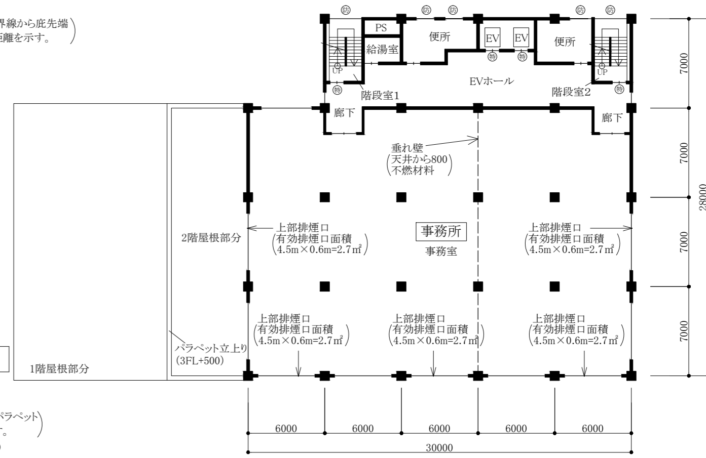
3～6階平面図
