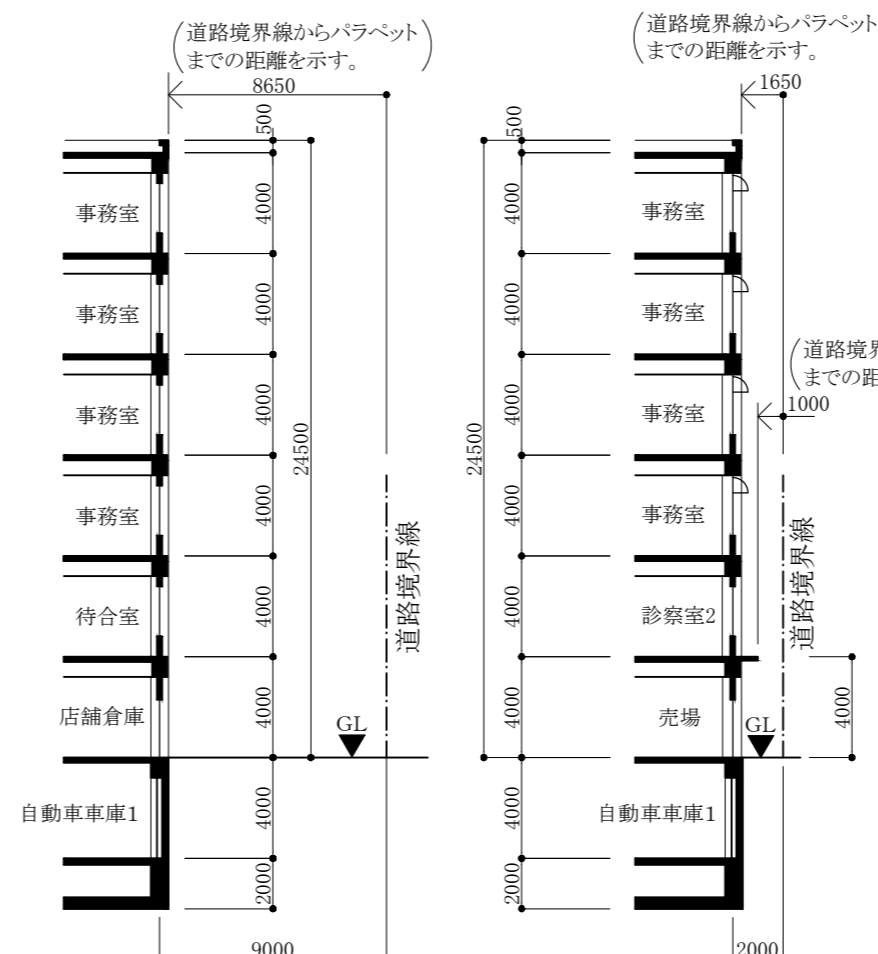
B-B' 断面図
