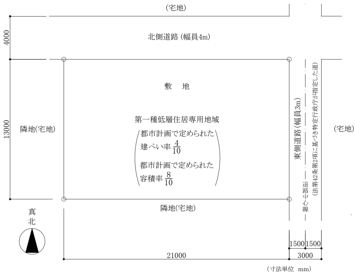
図1 (敷地平面図)
