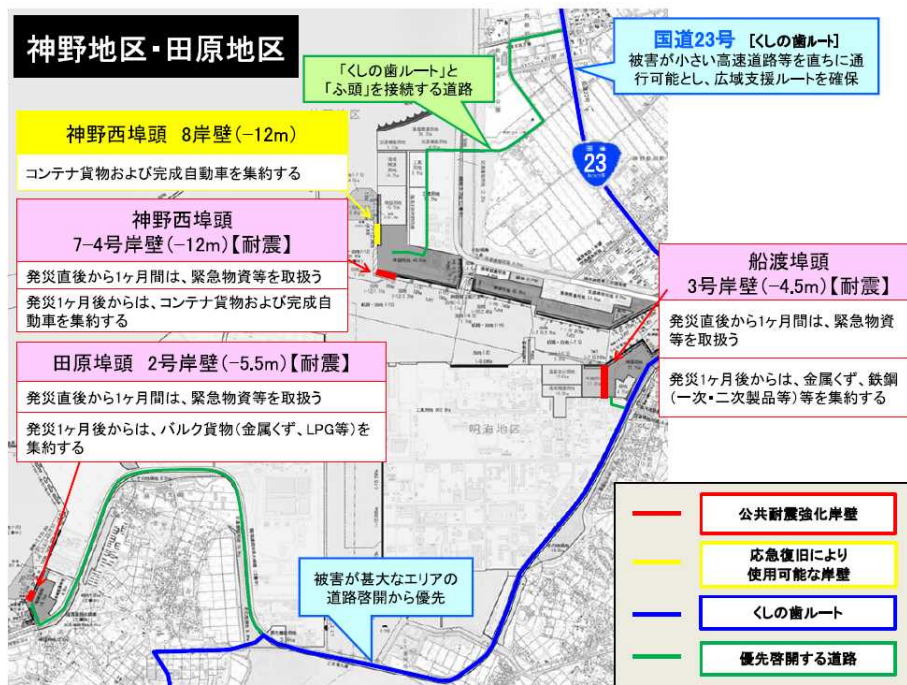
図－10 応急復旧優先岸壁および道路（案）（神野地区・田原地区）
