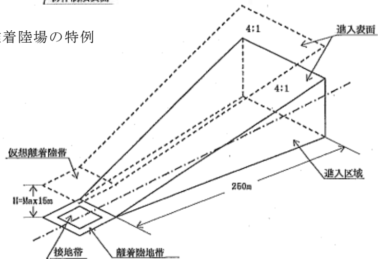
図－８－（２） 回転翼航空機の場合の進入区域、進入表面、仮想離着陸地の略図
