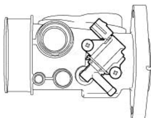
吸気ダクト
