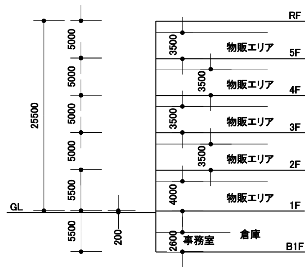
モデル建物（大規模物販店舗、5,000㎡） 階高及び天井高
