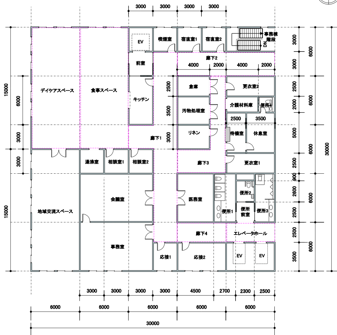
モデル建物（福祉施設、6,240㎡） 事務棟2階詳細図 1/200
