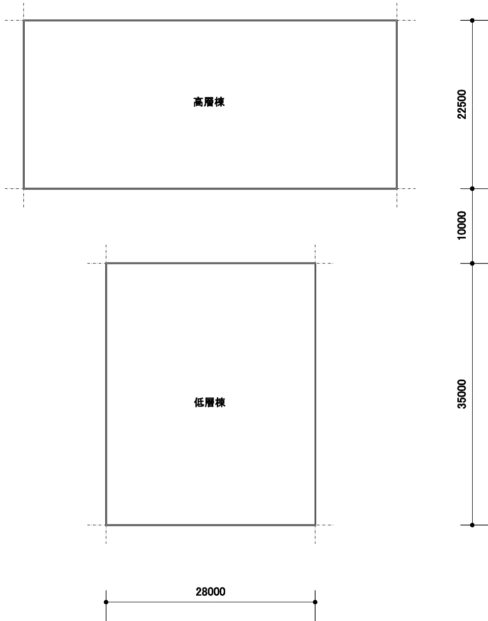
モデル建物（大学） 配置図 1/500
