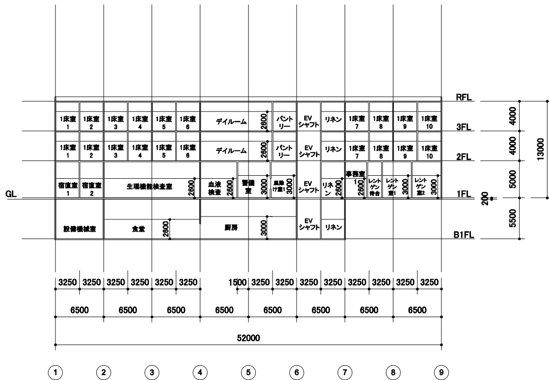
モデル建物（総合病院、5,000m²） A-A' 断面図 1/300
