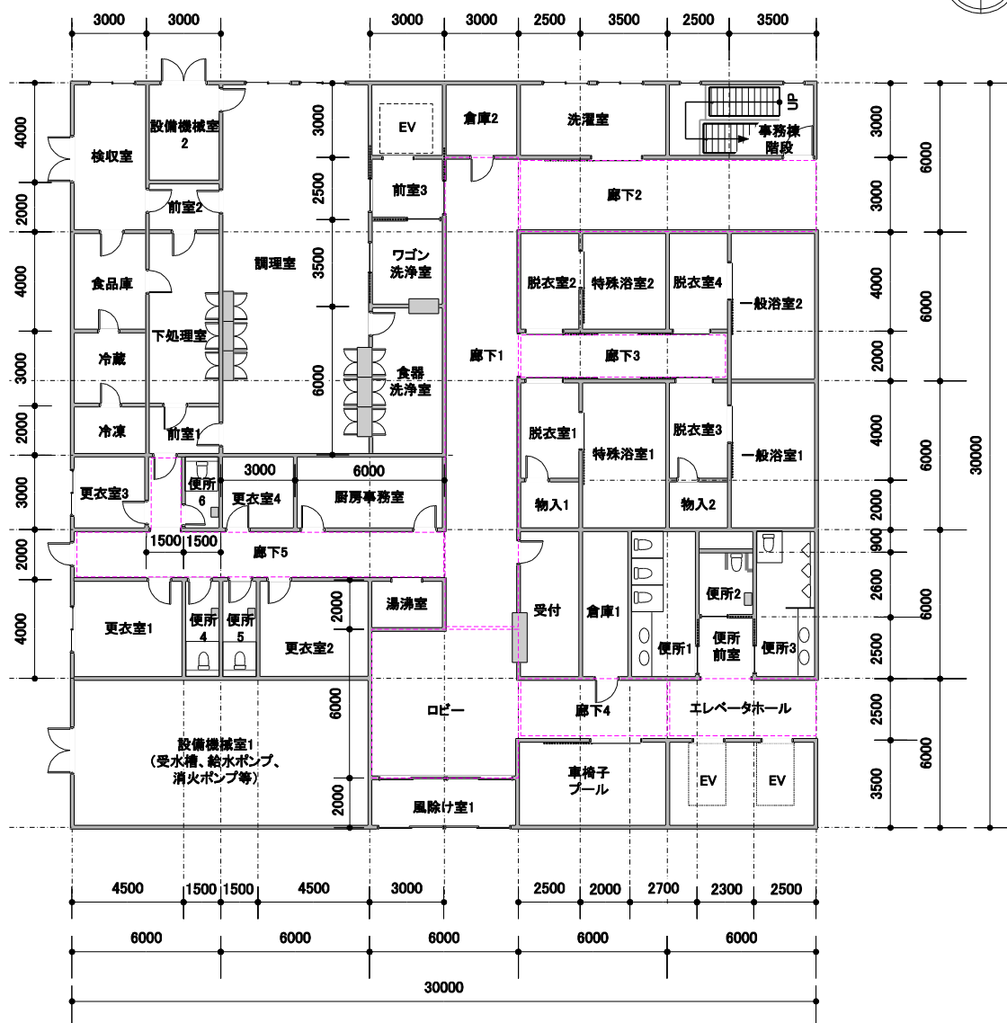
モデル建物（福祉施設、6,240㎡） 事務棟1階詳細図 1/200
