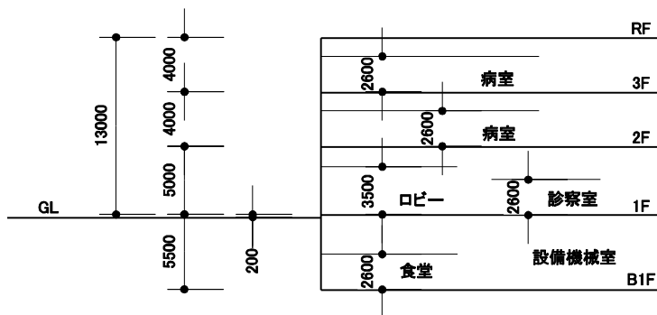
モデル建物（総合病院、5,000m²） 階高及び天井高
