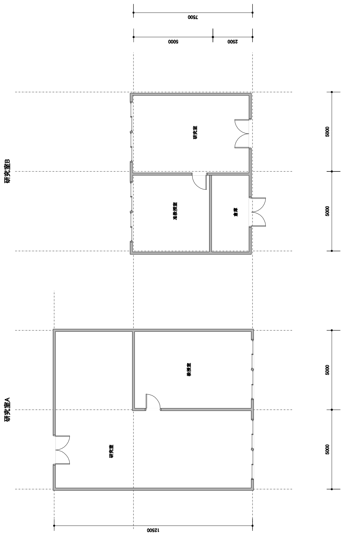
モデル建物（大学_高層棟、7,950㎡） 研究室平面詳細図 1/100
