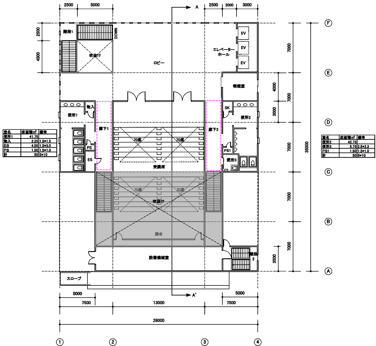
モデル建物（大学_低層棟、1,648.5㎡） 2階平面図 1/200
