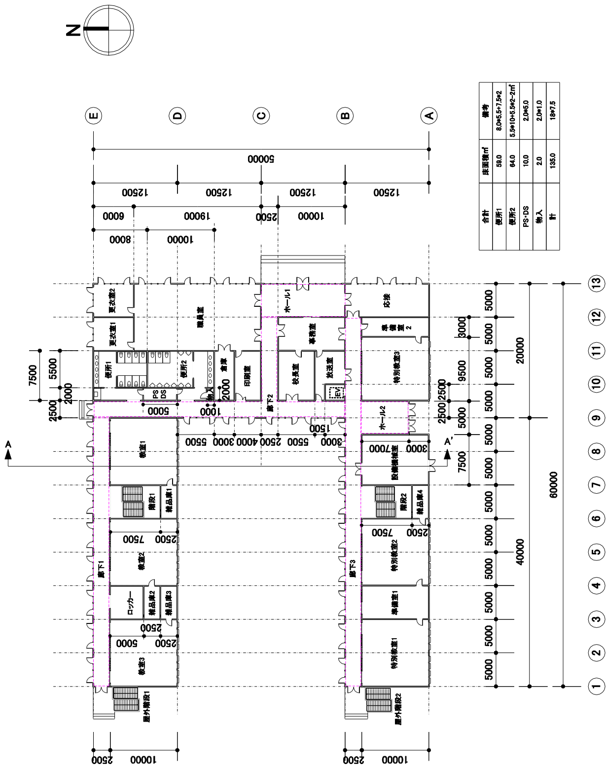
モデル建物（学校、5,000㎡） 1階平面図 1/500
