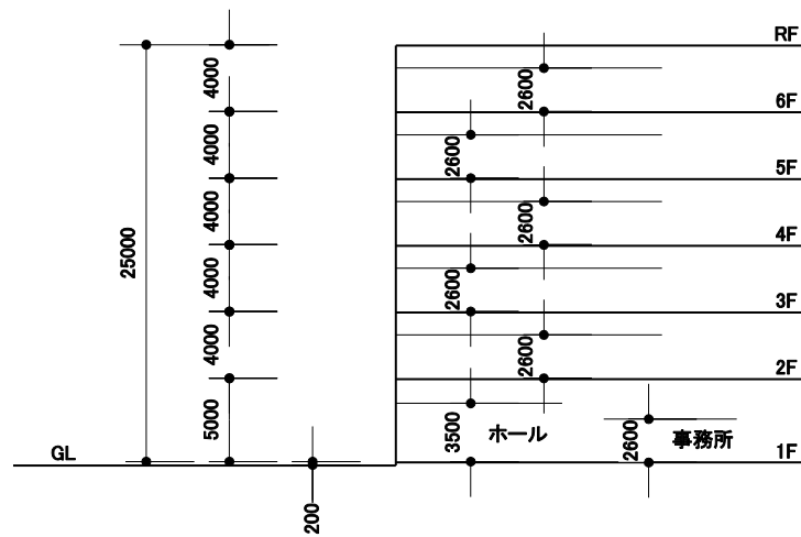
モデル建物（事務所、5,000㎡） 階高及び天井高
