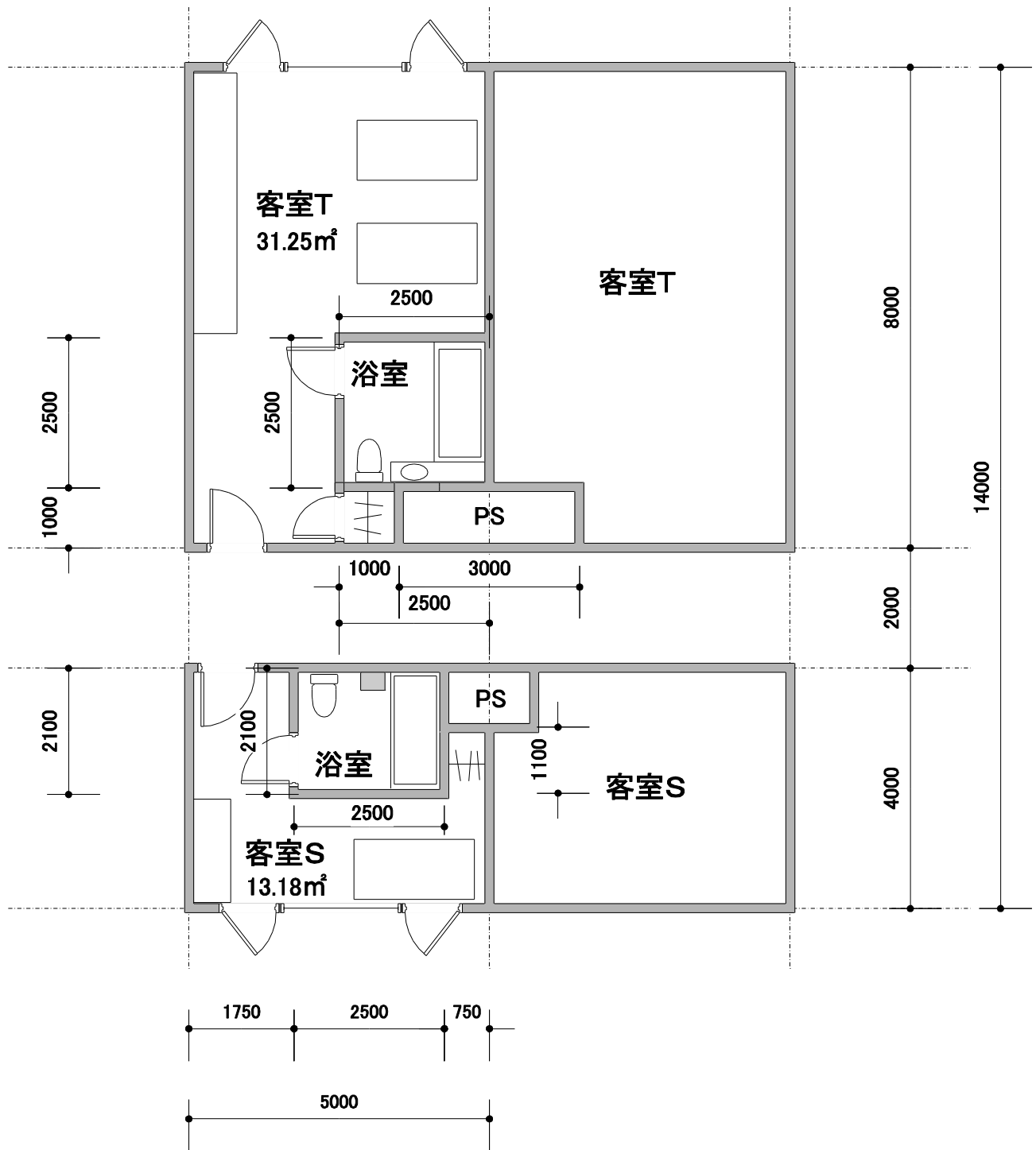
モデル建物（シティホテル、16,700m 2 ） 客室基準平面図 1/100
