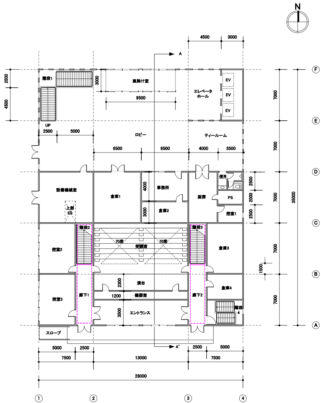
モデル建物（大学_低層棟、1,648.5m 2 ） 1階平面図 1/200
