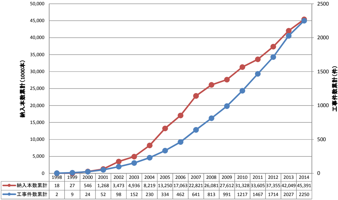
機械式鉄筋定着工法 納入本数、採用工事件数の推移
