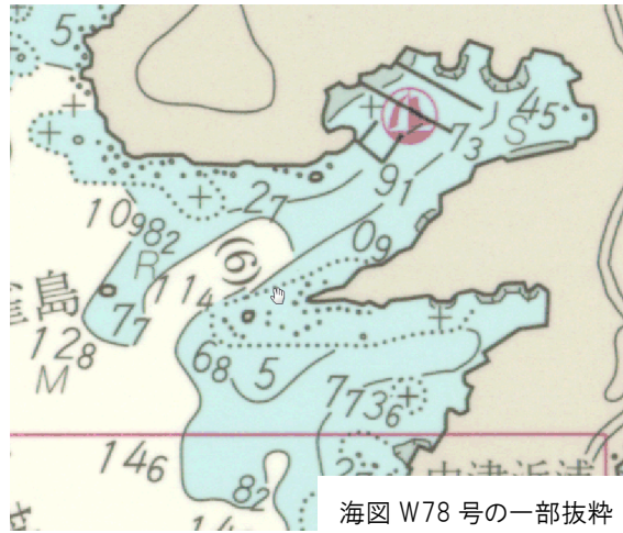
三重県 VOC 志摩ヨットハーバーの場合
