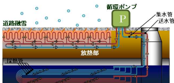
採熱部(熱交換施設)
