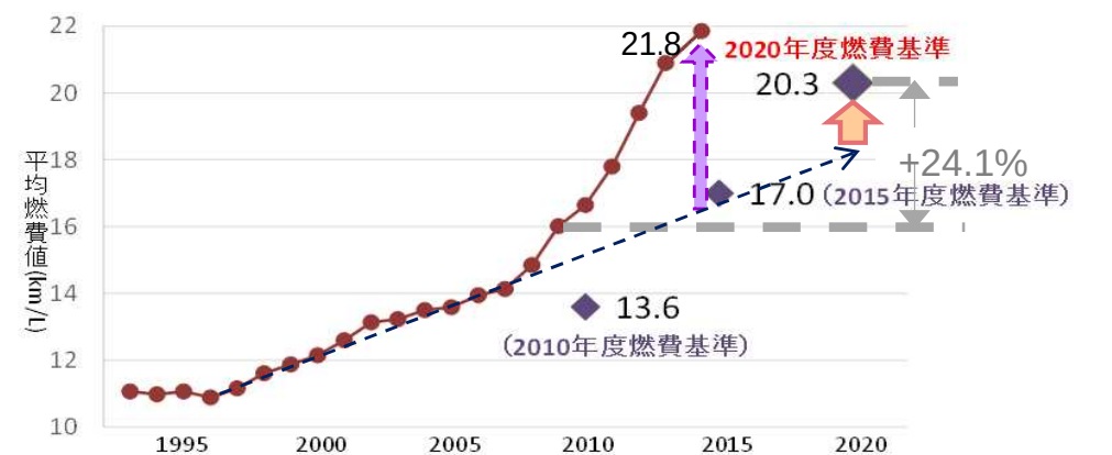
乗用車新車平均燃費と保有燃費の改善推移
