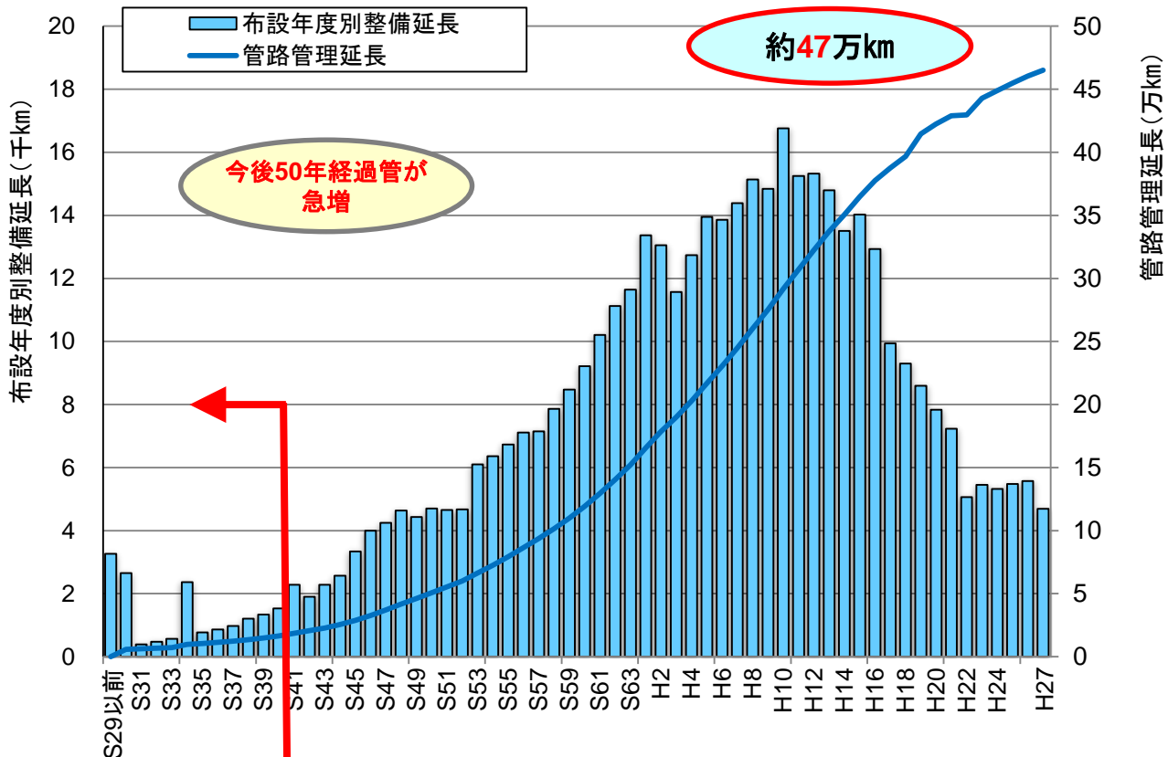
管路の年度別整備延長(H27末)
