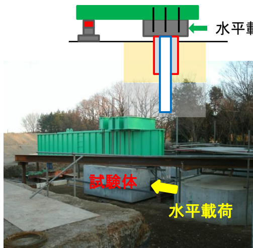
水平載荷試験実施状況
