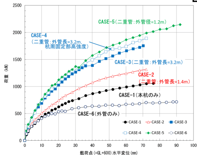
水平荷重—変位関係
