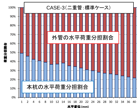
水平荷重分担率—変位関係
