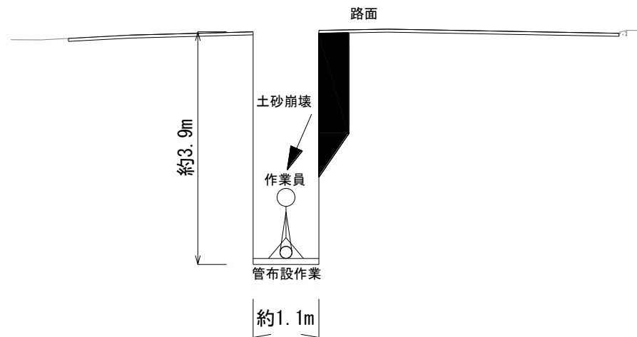
【断面図・状況図】
