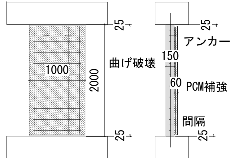
試験体
