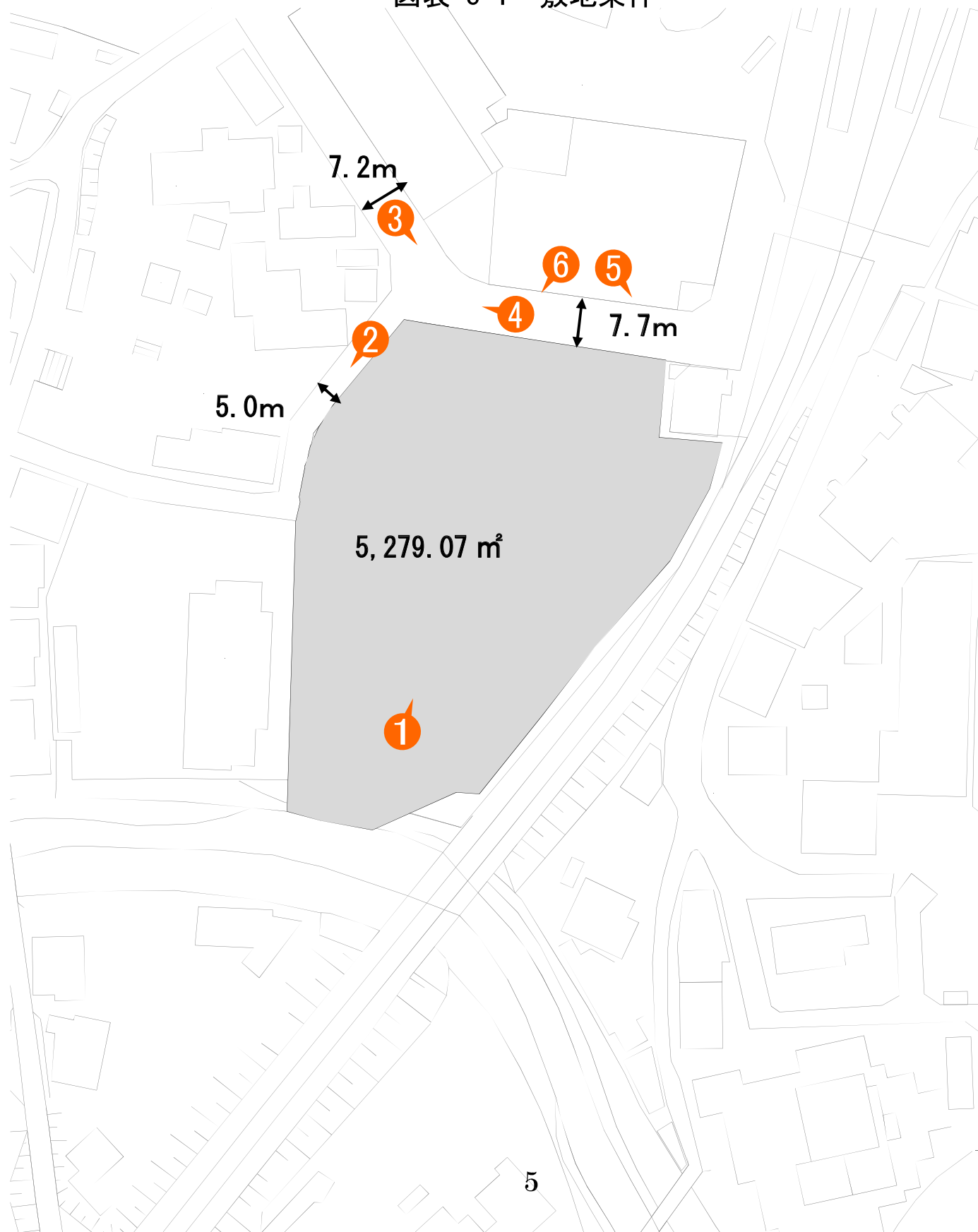
図表 3-1 敷地条件
