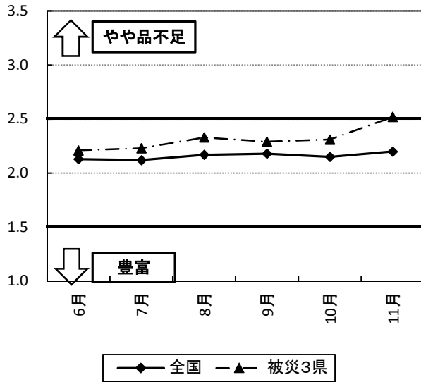
骨材(砕石)
