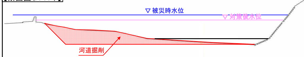
【断面図(A-A')】
