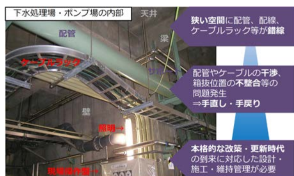
図 17 終末処理場・ポンプ場の内部の例
