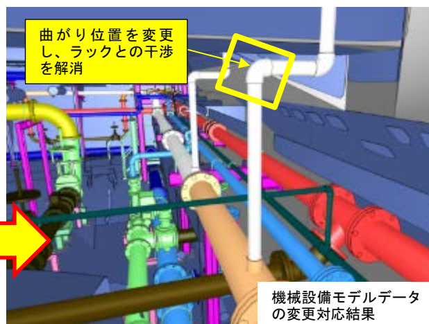
空気が管とラックとの干渉を解消（施工段階）
