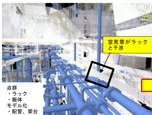
空気が管とラックの干渉チェック（施工段階）
