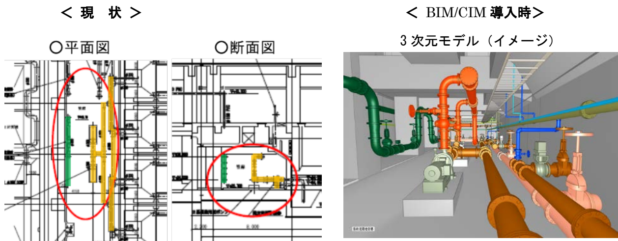
図 13 BIM/CIM のイメージ図
