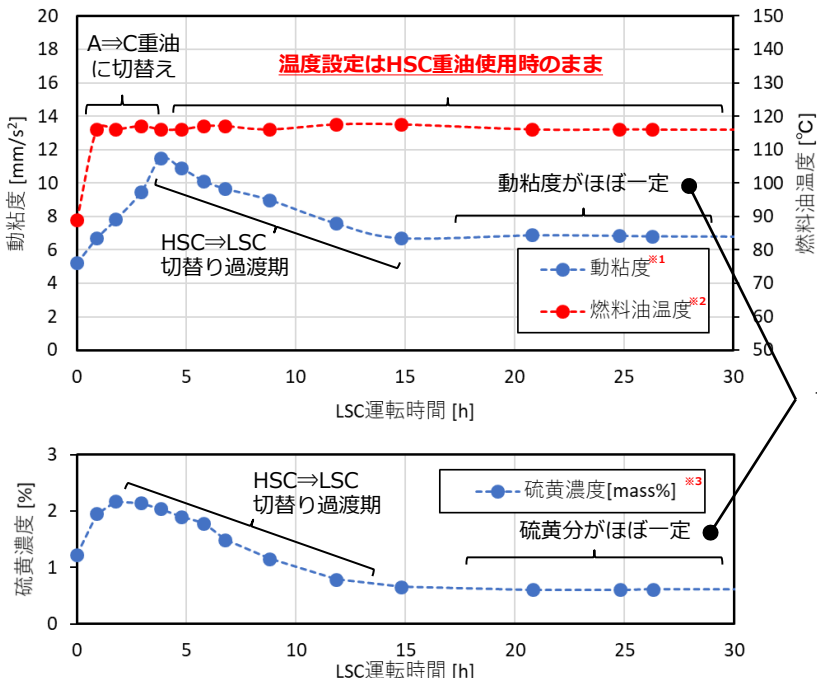
ビスコン無い場合の性状の推移例 (温度調整装置により温度を一定に調整)
