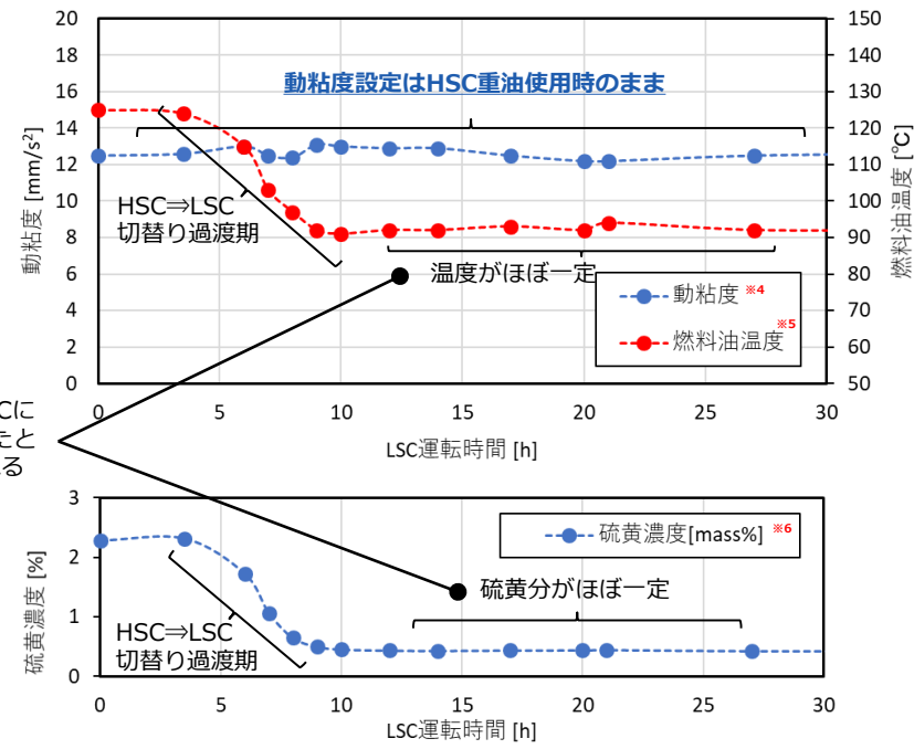
ビスコンが有る場合の性状の推移例 (粘度調整装置により動粘度を一定に調整)
