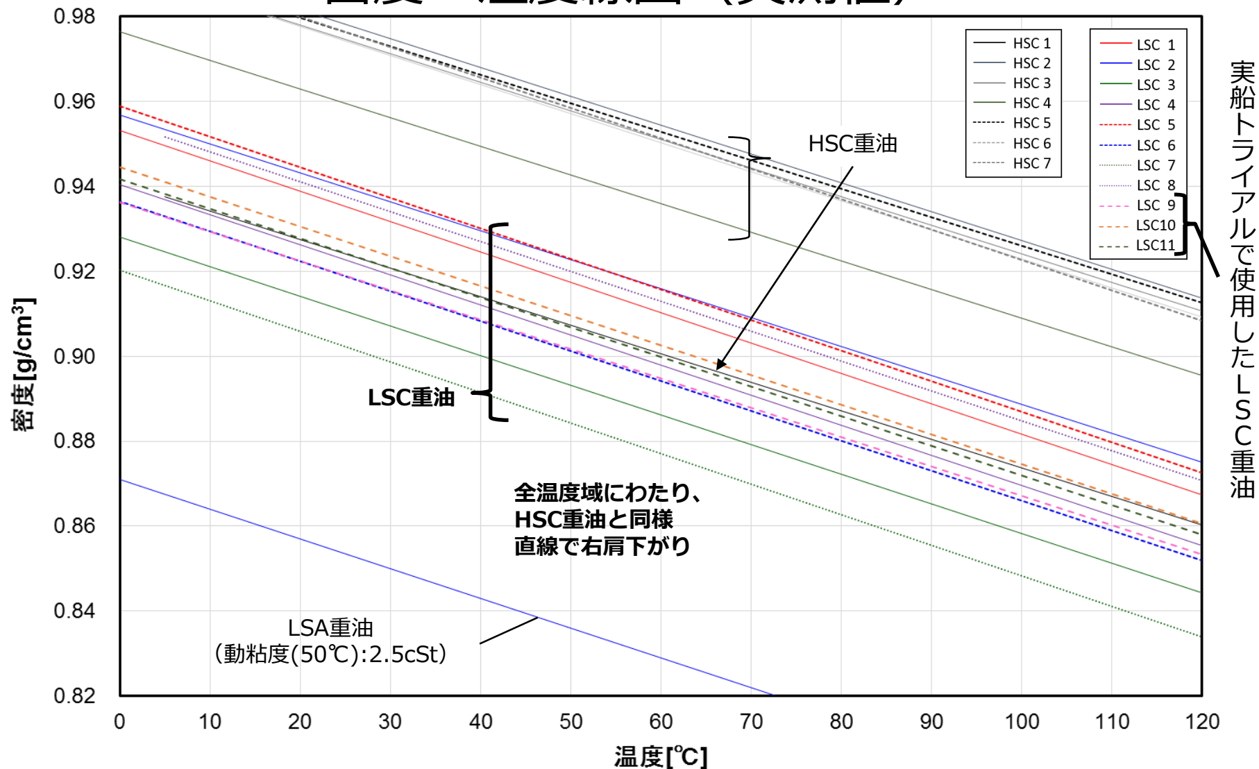
密度－温度線図（実測値）
