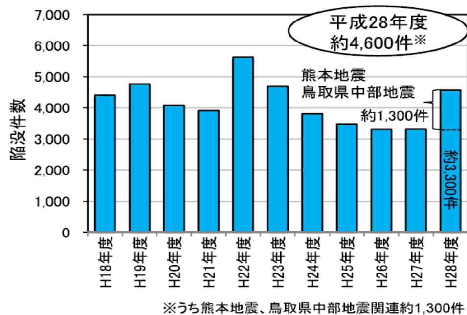
参考 3－8－4 下水道管路施設に起因した道路陥没件数の推移（平成 28 年度末）
