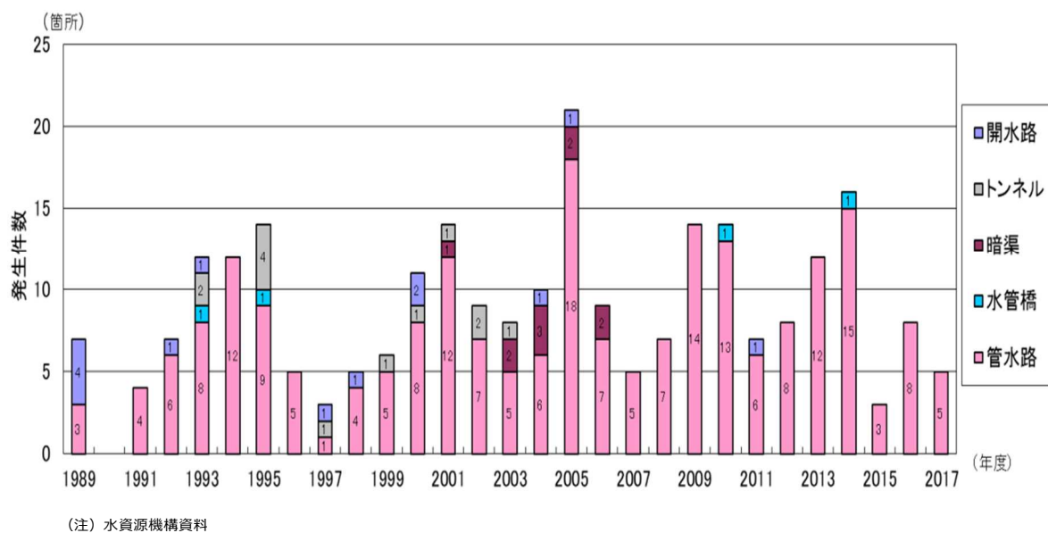
参考 3-8-5 水資源機構の施設における漏水事故発生件数の推移
