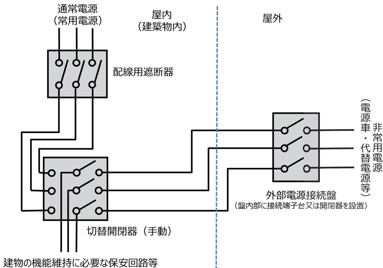
標準的な外部電源接続盤にかかる回路及び機器構成
