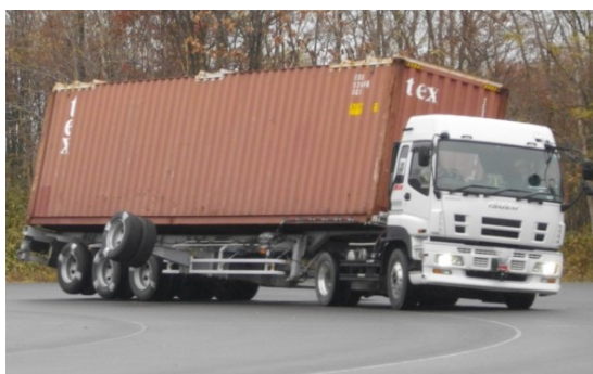
図7 横転限界時のトレーラーの状態
