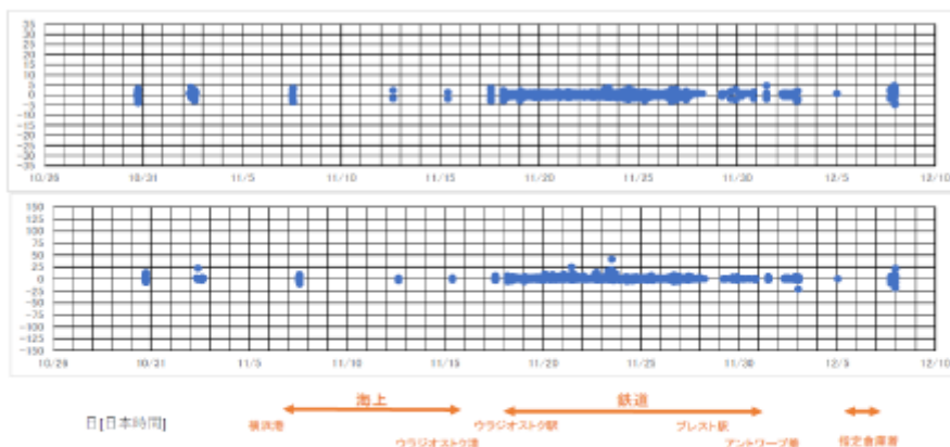
図Ⅲ. 横浜～アトワープ間の振動・衝撃値（Y軸／前後方向）
