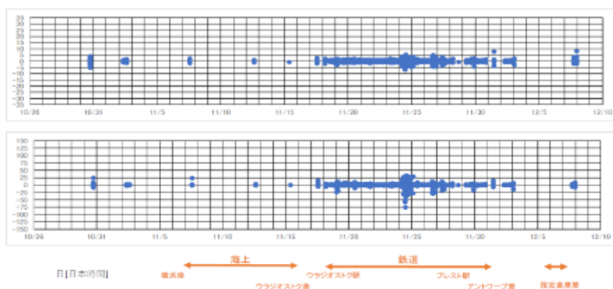
図Ⅱ. 横浜～アントワープ間の振動・衝撃値（X 軸／前後方向）
