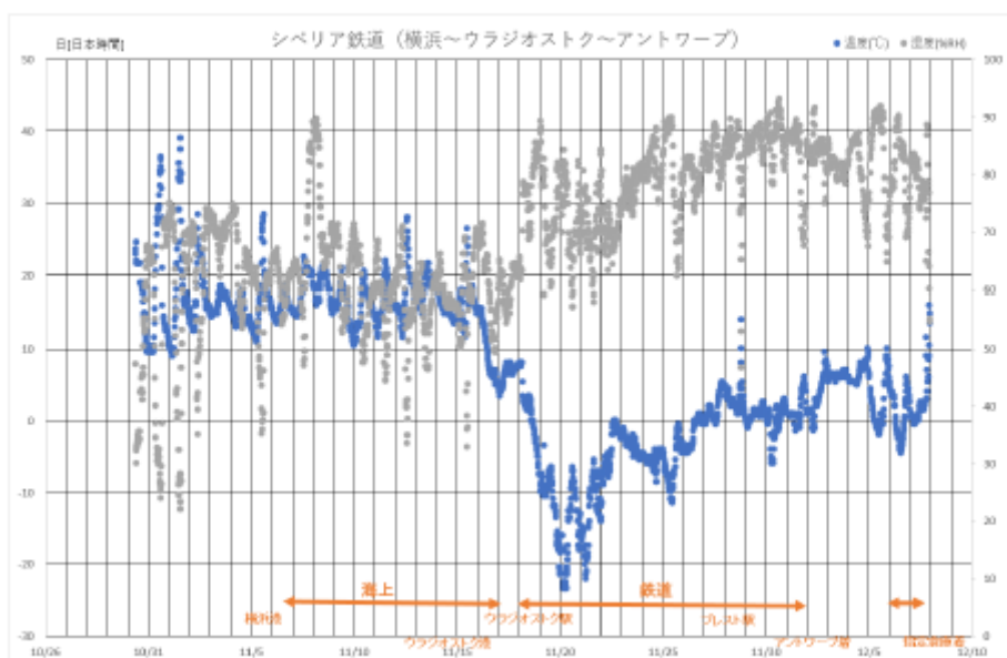
図V. 横浜～アントワープ間の温湿度推移
