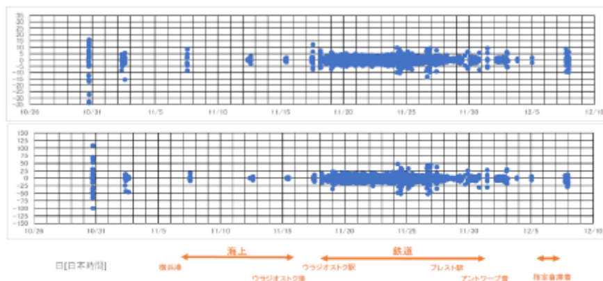
図Ⅳ. 横浜～アトワープ間の振動・衝撃値（Z軸／前後方向）
