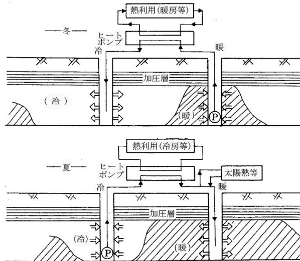
図2 地下水の熱利用システムの例
