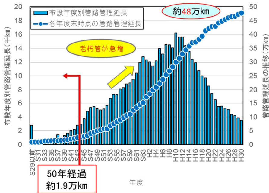
参考 3－8－3 下水道管路施設の年度別管理延長（平成 30 年度末）
