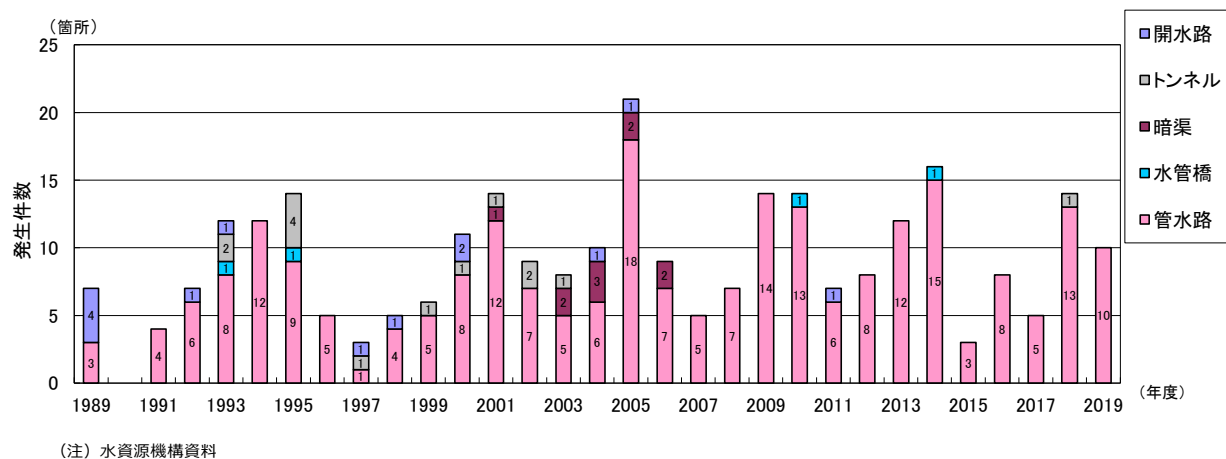
参考 3-8-5 水資源機構の施設における漏水事故発生件数の推移
