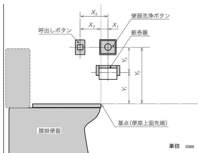
参考 操作部及び紙巻器の配置及び設置寸法（JIS S 0026）
