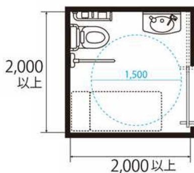
ライニングなしの場合
