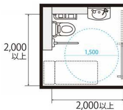
ライニングありの場合
