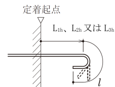
フックありの定着の長さ
