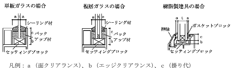
図 16.14.1 ガラス溝
