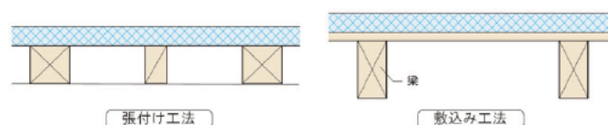
外張断熱工法の種類
