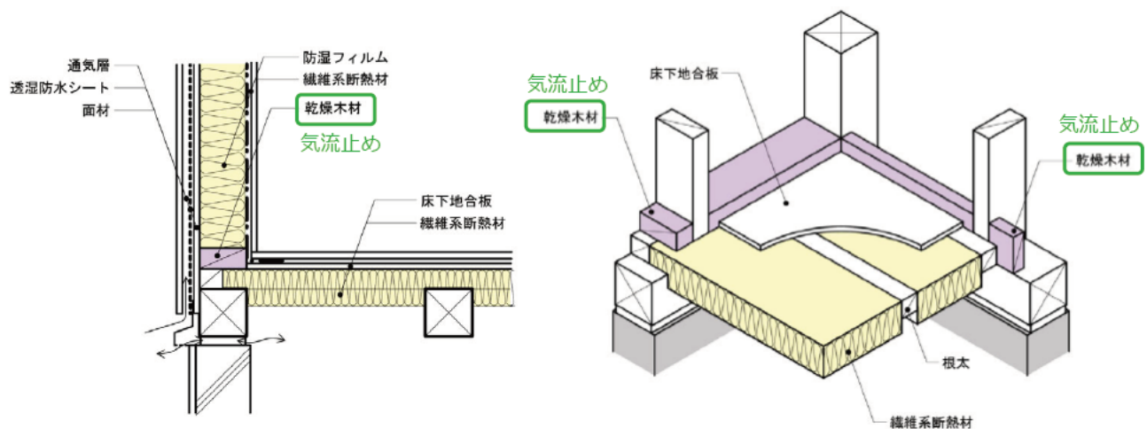
乾燥木材を使った気流止めの方法
