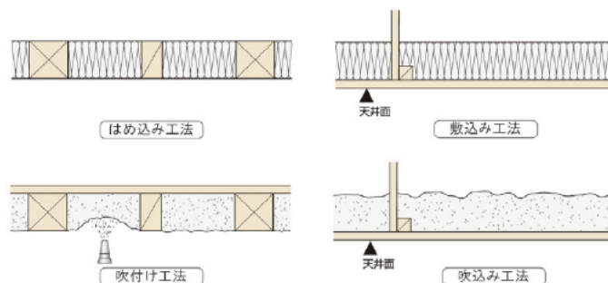
充填断熱工法の種類
