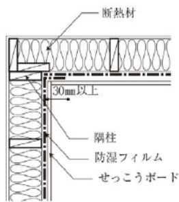
隅角部 (例)
