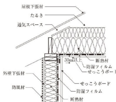
外壁と最上階の天井の 取合い部 (例)
