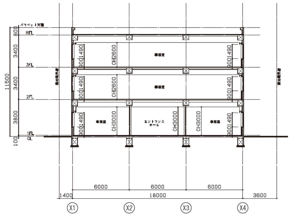
B断面図
