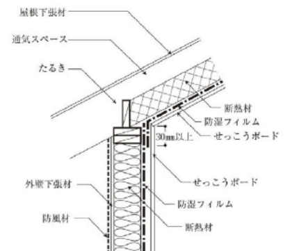
外壁と屋根の 取合い部 (例)
