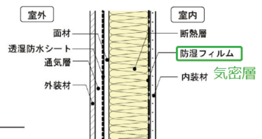
気密層の設置位置 (繊維系断熱材の場合)
