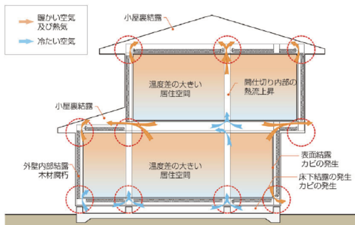
木造軸組構法の断熱上の問題点
