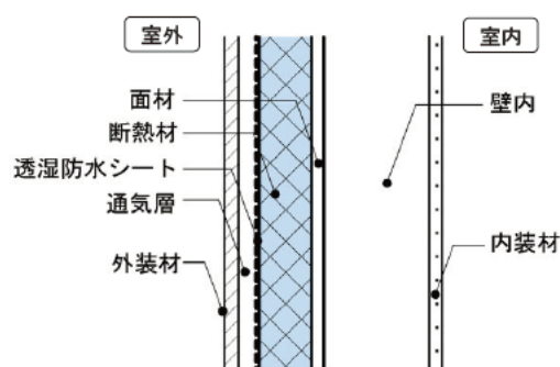
外張断熱工法の外壁の断面構成
