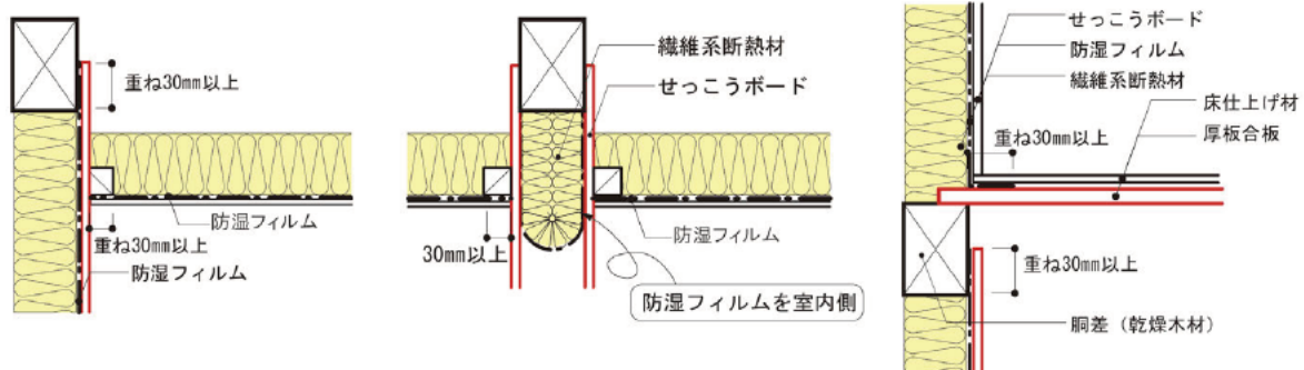
天井と外壁・間仕切り壁の気流止め
