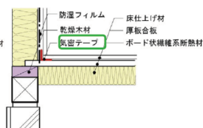
気密テープで押さえる方法
