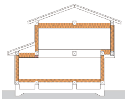
充填断熱工法
