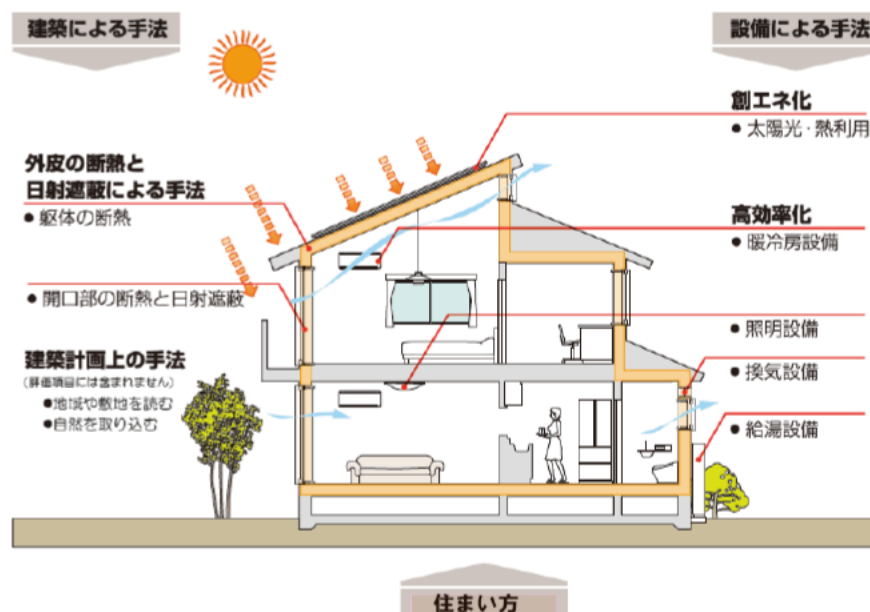
省エネルギー化のための手法（イメージ図）
