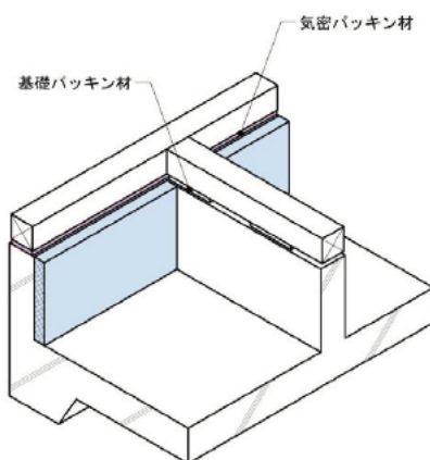
基礎内側断熱
