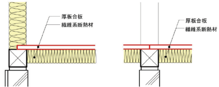
壁が充填断熱の場合
