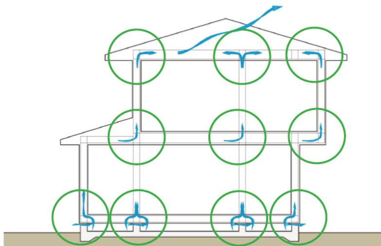
気流止めを施工しない場合に起こる壁内気流の例
