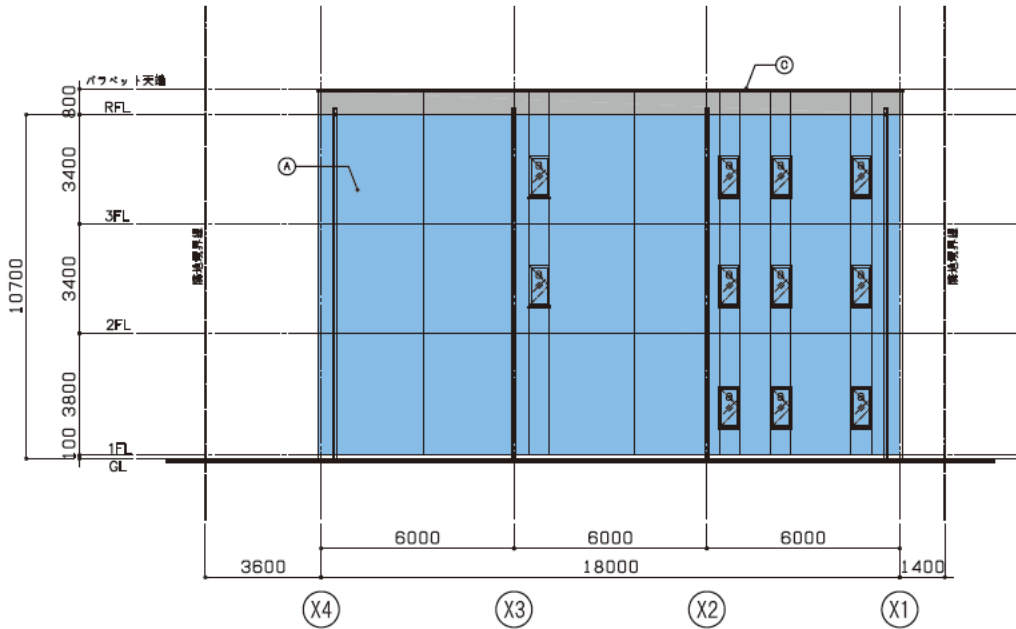
北側立面図
