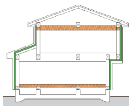
充填断熱工法 + 外張断熱工法
