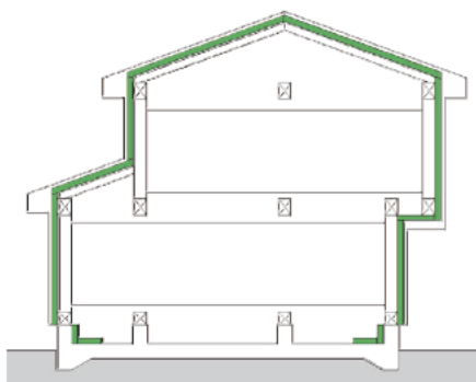
外張断熱工法
