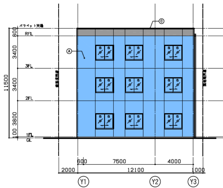
東側立面圖
