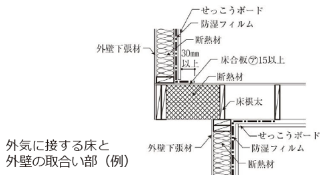
床と外壁の取合い部（例）
