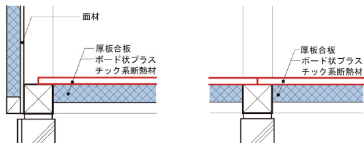
壁が外張断熱の場合
