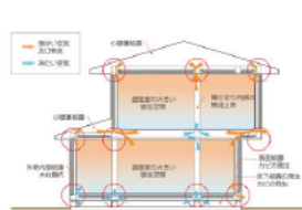
木造軸組構法の断熱上の問題点
