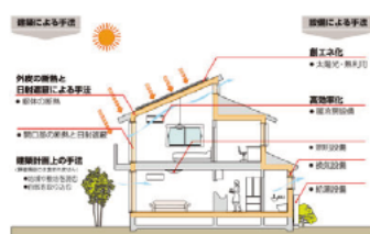
図 1.2.3 省エネルギー住宅のための手法（イメージ図）
