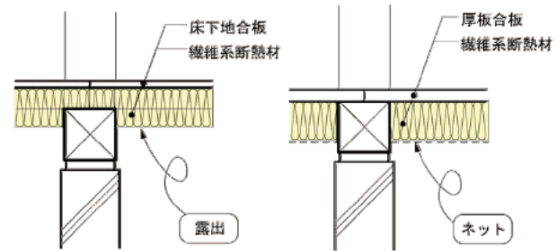
床の防湿フィルムを省略できる場合
