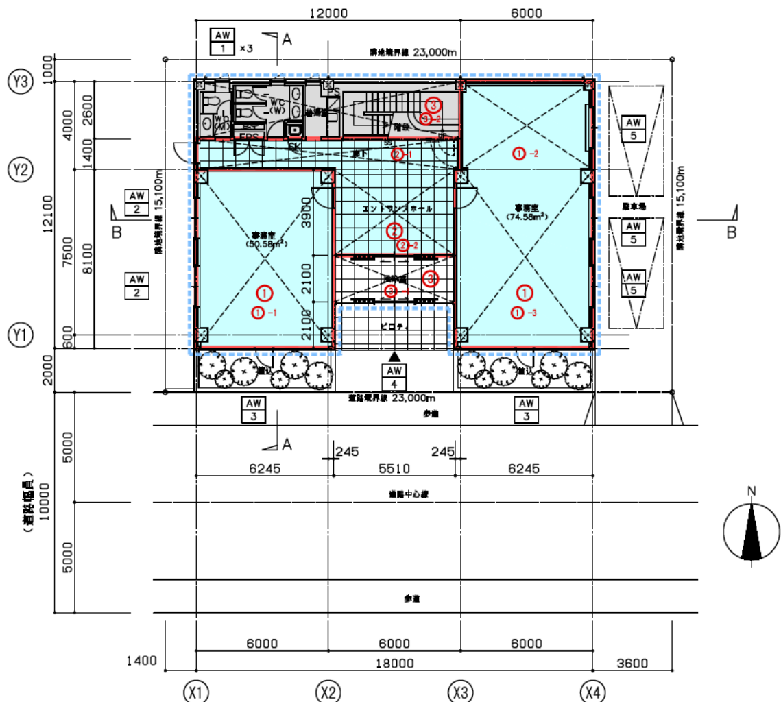
配置図・1階平面図
