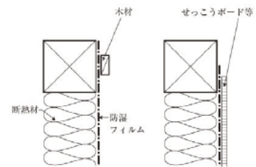
防湿フィルムの端部の押さえ
