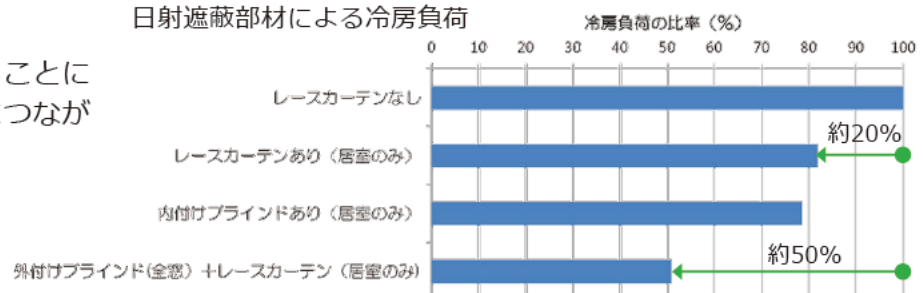
日射遮蔽部材による冷房負荷
