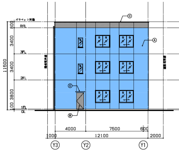
西側立面圖
