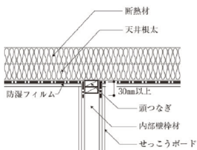
4～7地域 内壁の頭つなぎに天井の防湿フィルム を30mm以上留め付ける
