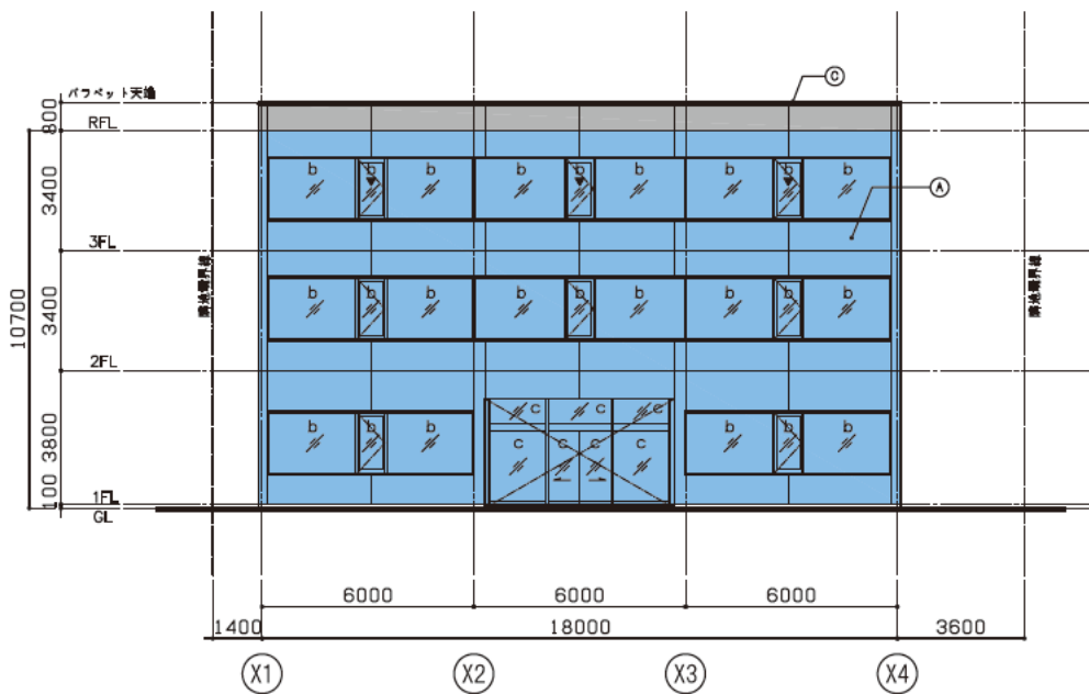
南側立面図
