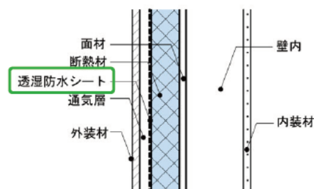
外張断熱工法 (発泡プラスチック系断熱材使用)
