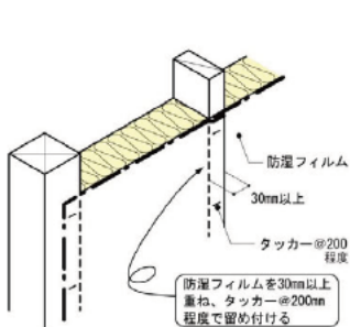
図 5.3.6 防湿フィルムの重ね
