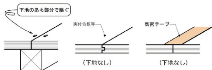
床の気密の取り方
