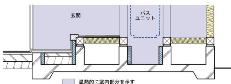
床断熱の場合の床下の断面
