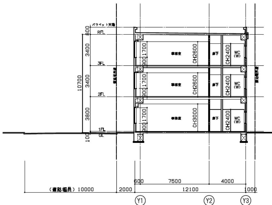
A断面図
