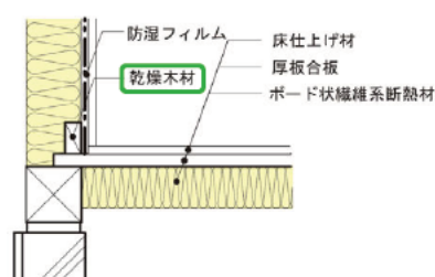
乾燥木材で押さえる方法
