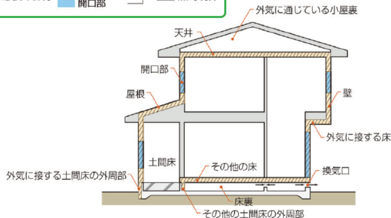
熱的境界
