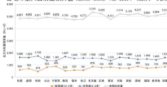
各地の全天日射量積算値 (暖房期、冷房期、年間/2019年 気象庁データより作成)
