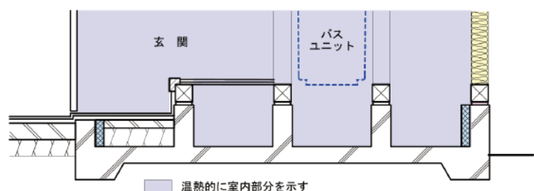
基礎断熱の場合の床下の断面
