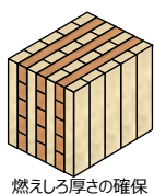
燃えしろ厚さの確保
