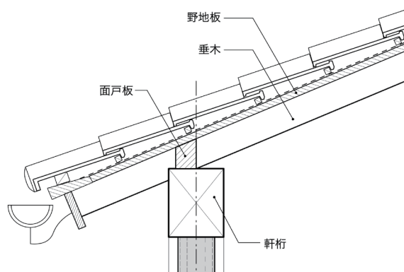
図 2-11 面戸板現し
