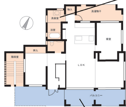
図 3-4 バッファゾーンによる平面構成
