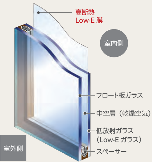
Low-E 二層複層ガラス
