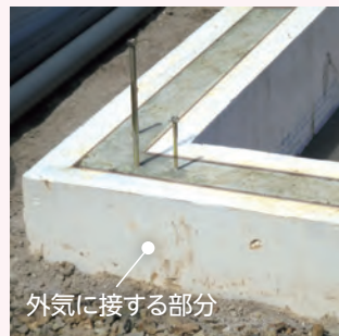
写真は 充填断熱 + 付加断熱工法
