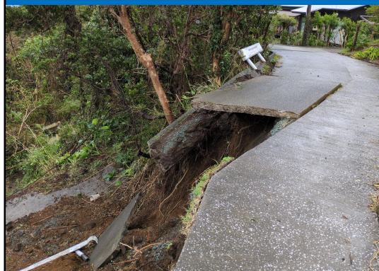
被災状況調査(東京都八丈町)
