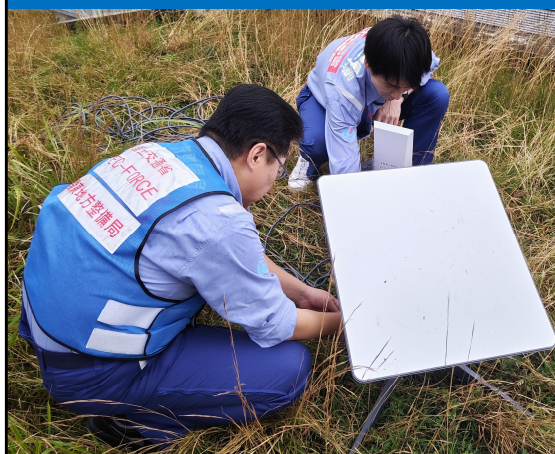
衛星インターネット装置(東京都八丈町)
