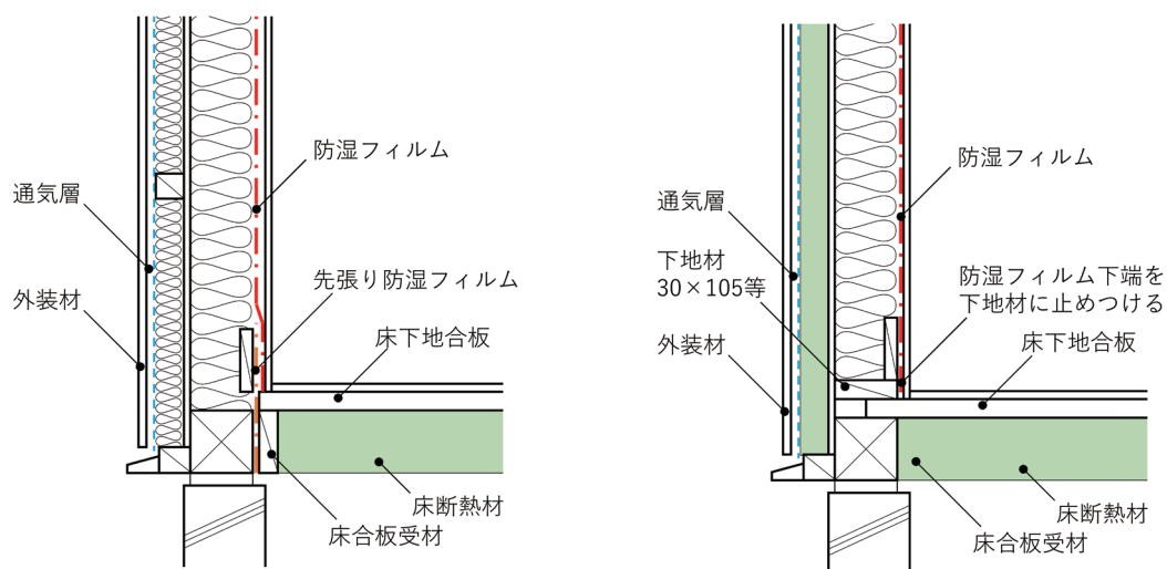
(a) 先張り防湿フィルムによる方法
