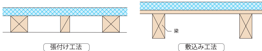
図 3.1.6 外張断熱工法の種類
