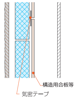
(b) 断熱材の室内側の構造用合板等の目地を気密テープで処置する
