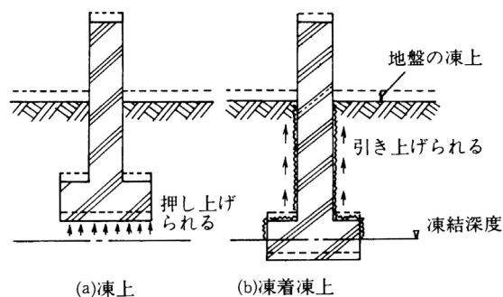
図 2.1.1 凍上の原因（主なもの）
