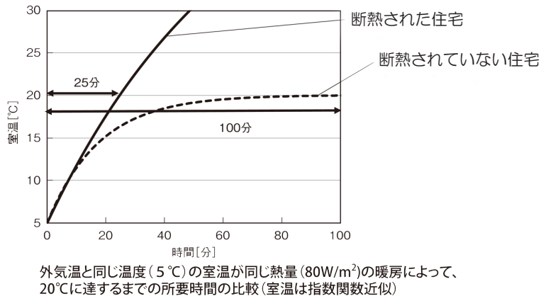
図 2.2.11 暖まるまでの所要時間 出典：HEAT20「設計ガイドブック」
