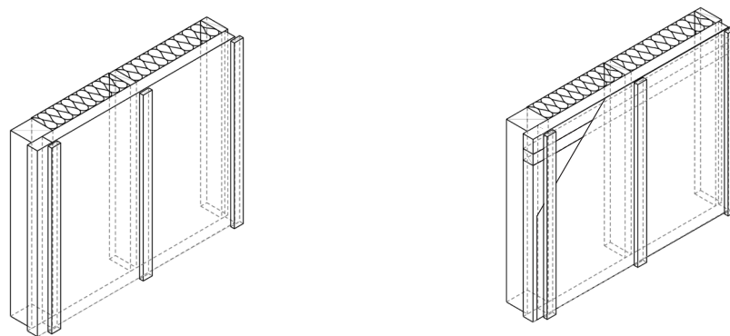
(a) 発泡プラスチック系断熱材の付加断熱施工方法
