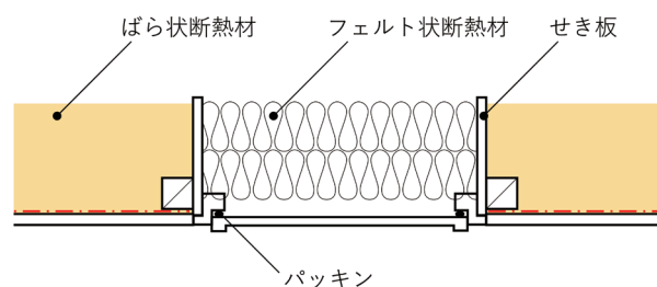
図 5.5.3 ばら状断熱材用の作業口まわりの気密施工例
