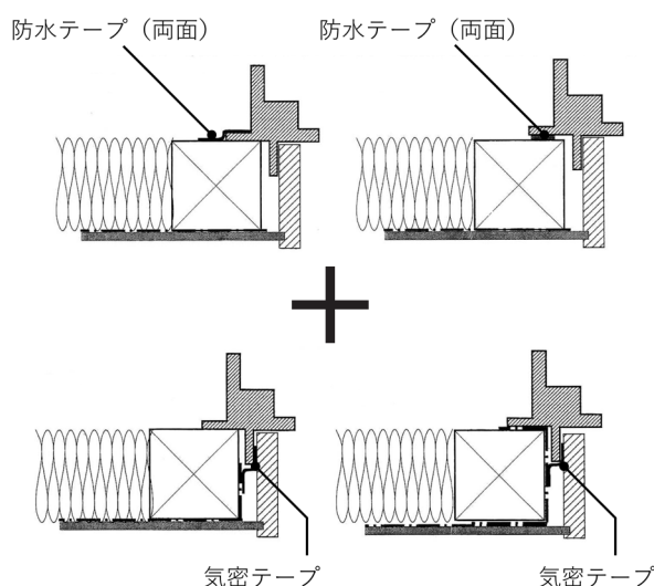
(a) サッシの外側からシールする場合
