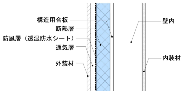
図 3.2.3 外張断熱工法
