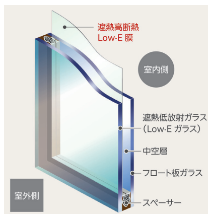
図 3.3.4 Low-E 複層ガラス [日射遮蔽型]
