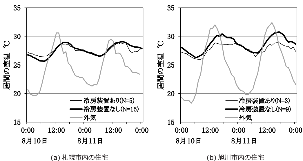
図 2.3.1 夏の温度推移
