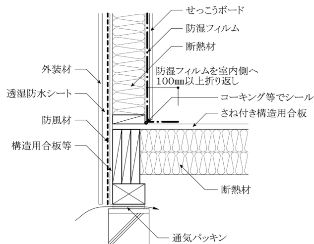
(b) 根太間断熱の場合
