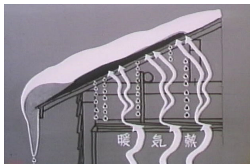
図 2.1.2 すがもれの原因
