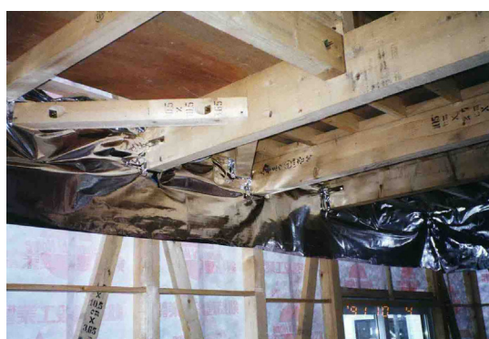
写真 5.2.2 先張り防湿フィルムの施工例 1
