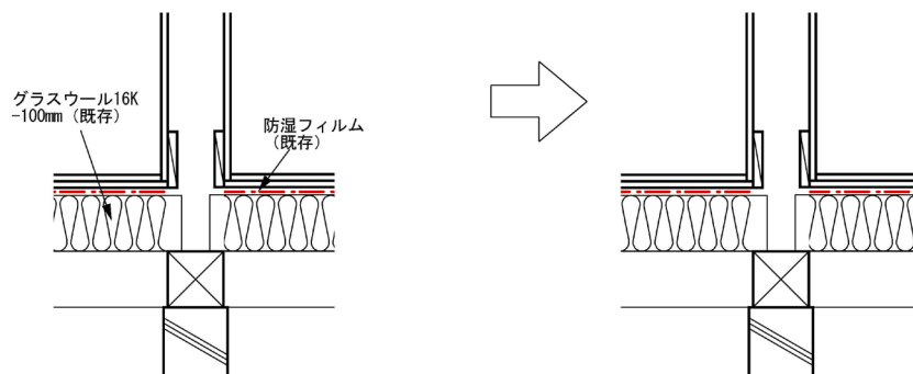
図 8.2.6 間仕切壁と１階床の取合い部（基礎断熱工法の場合）
