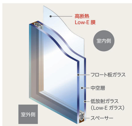
図 3.3.3 Low-E 複層ガラス [日射取得型]
