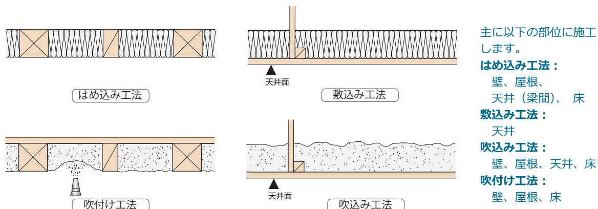
図 3.1.5 充填断熱工法の種類
