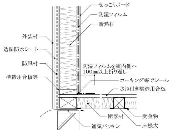
(a) 大引き断熱の場合
