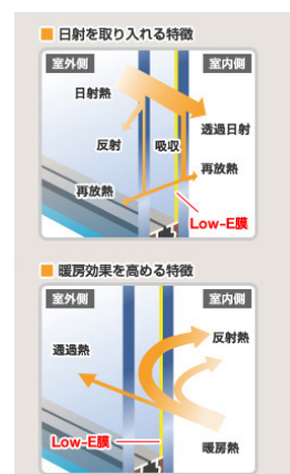
図 3.3.3 Low-E 複層ガラス [日射取得型]
