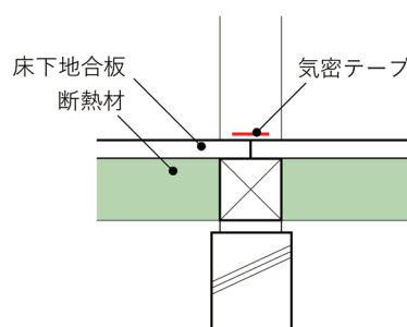
図 5.5.1 柱下部が防湿フィルムを貫通する部分の施工例
