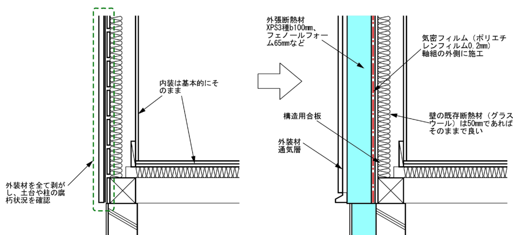
図 8.2.16 外壁と1階床の取合い部
