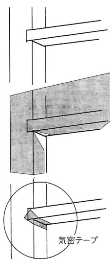
(c) サッシ内側からシールする場合
