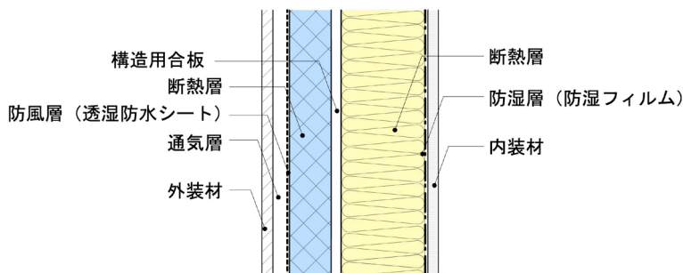
図 3.2.4 付加断熱工法
