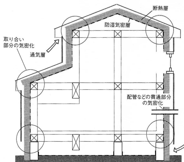
図 5.3.1 外張断熱工法
