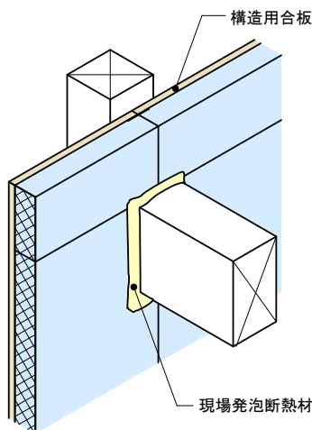
図 5.3.22 貫通部の断熱補強
