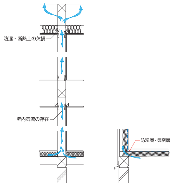
図 3.3.18 気流止めを施工しない場合に起こる壁内気流の例
