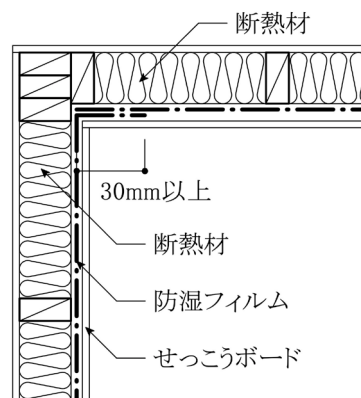
図 6.1.4 隅角部
