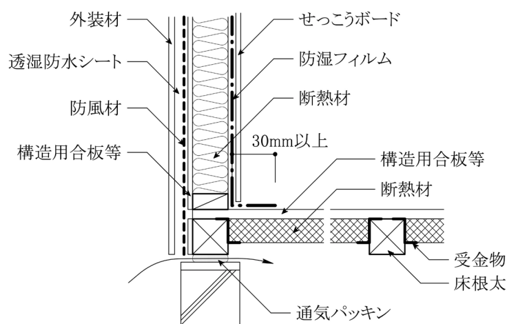
図 6.1.2 床と外壁の取合い部
