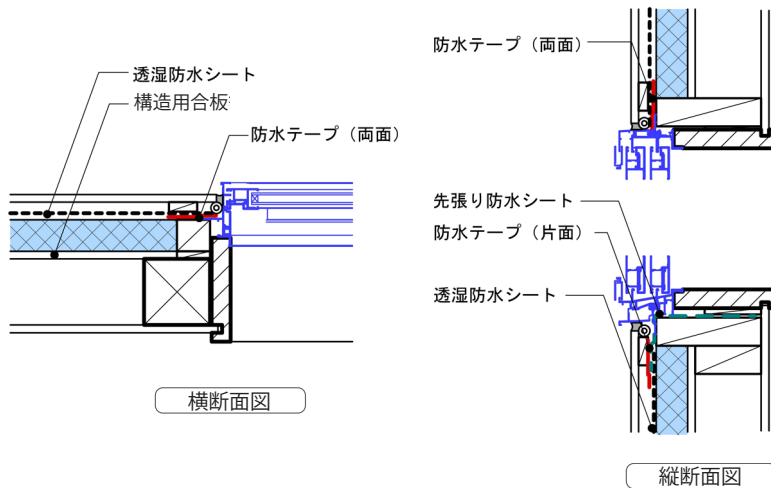
図 5.4.4 外張断熱工法の開口部まわり
