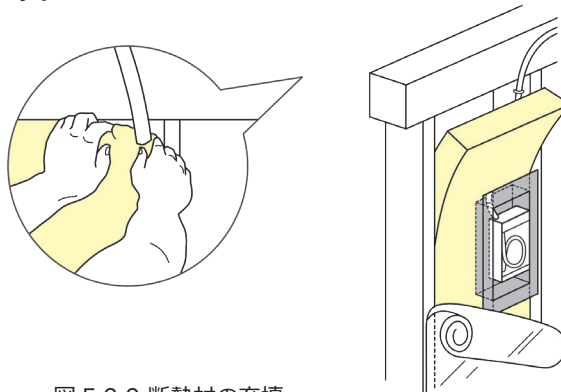
図 5.9.9 断熱材の充填
