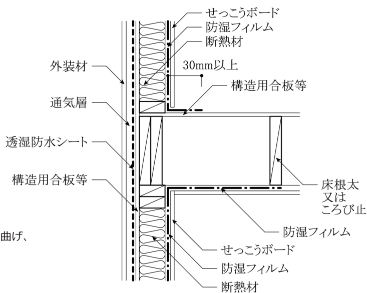
図 6.1.6 その他の階の床と外壁の取合い部
