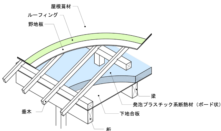
図 5.6.8 桁上断熱
