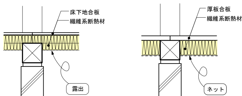
図 5.2.3 床の防湿フィルムを省略できる場合
