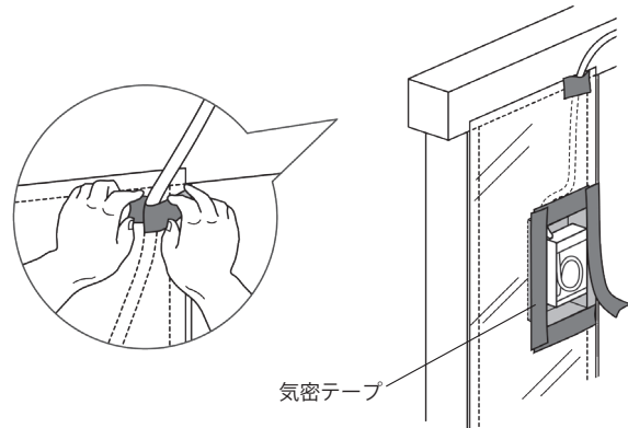
図 5.9.11 気密テープの施工
