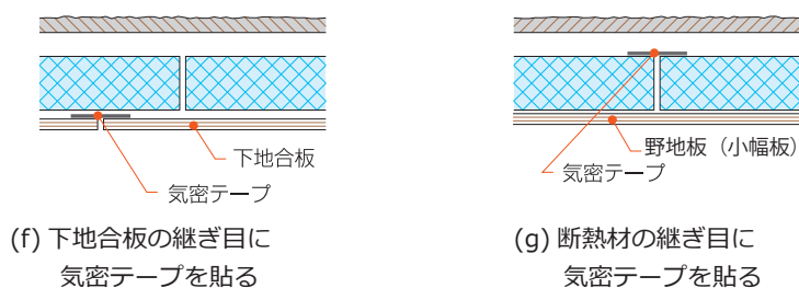
図 3.3.15 外張断熱工法における屋根の気密層の確保の方法
