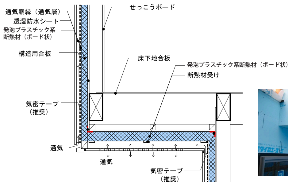
図 5.2.16 外壁が外張断熱工法の軒天断熱
