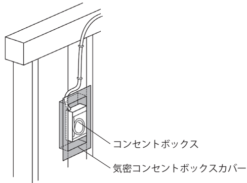
図 5.9.7 コンセントボックスの取付け
