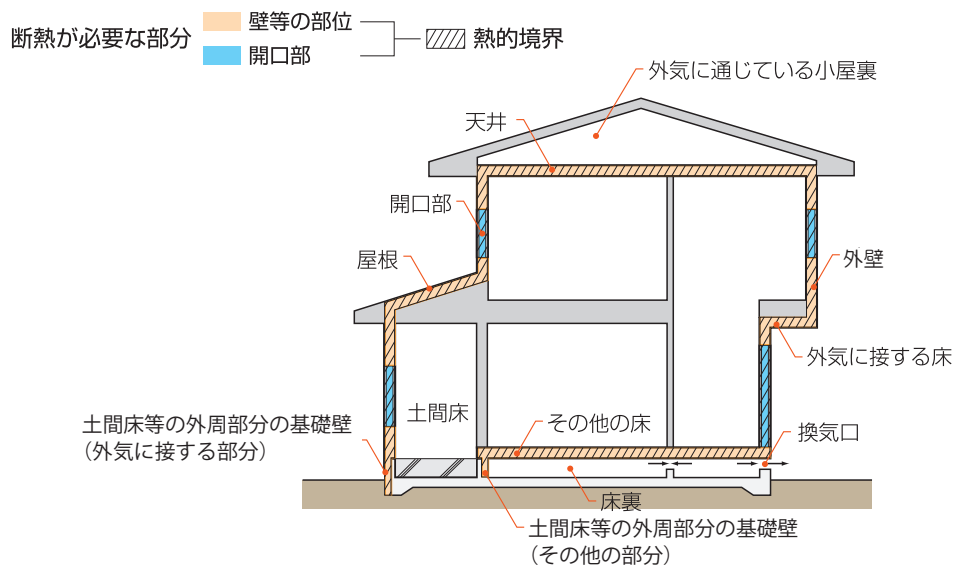
図 3.3.1 熱的境界
