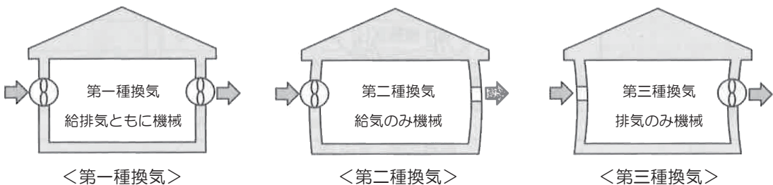
図 3.5.3 換気方式の種類
