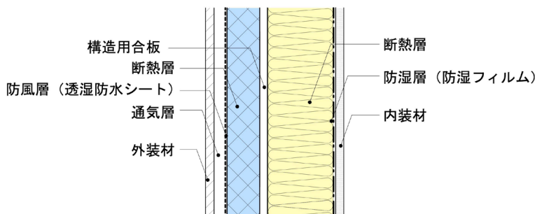
図3.3.4 付加断熱工法
