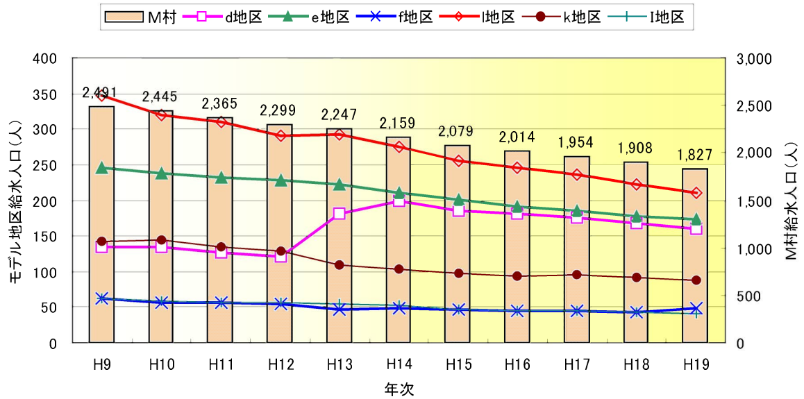
図 7.3.1 モデル地区の給水人口
