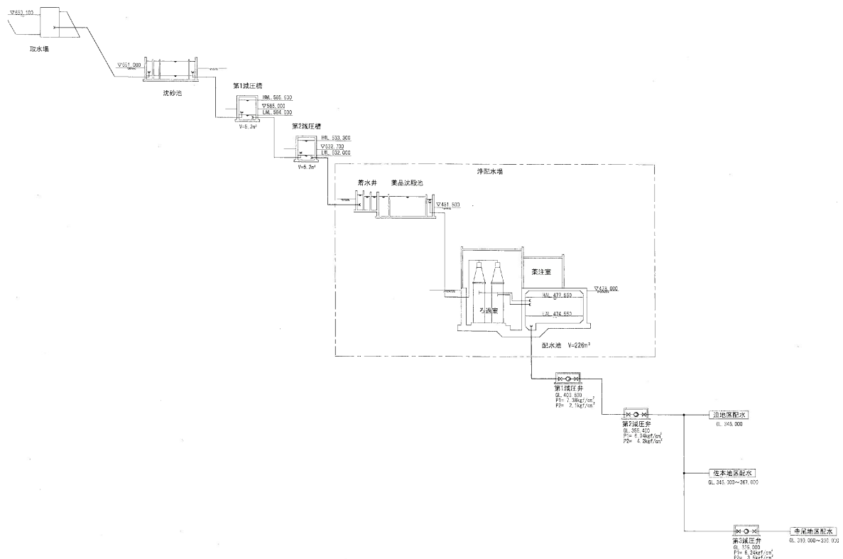
図 7.3.3 d地区水位関係図
