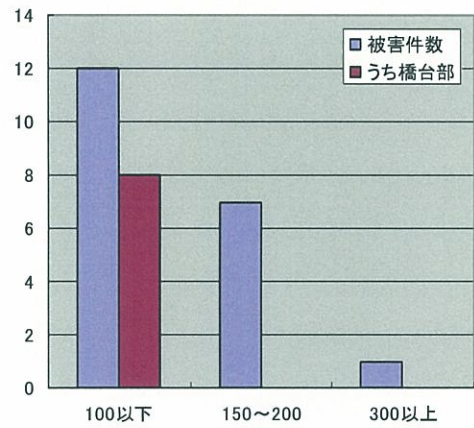
図 5.14 橋台取合部の被害件数
