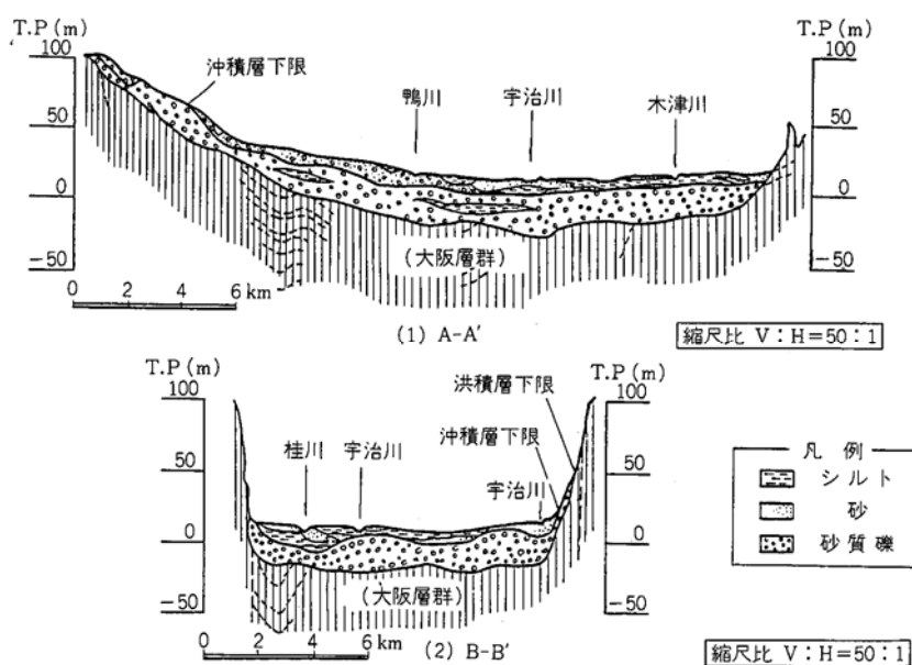
図一3.2.6 地質断面図 (出典:地下水要覧)
