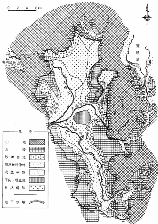
図一3.2.4 京都盆地の地形分類 (出典:地下水要覧)
