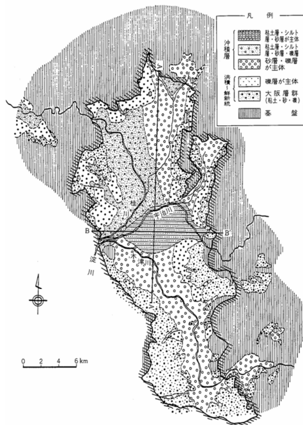
図 3.2.5 京都盆地の地質概要 (出典:地下水要覧)
